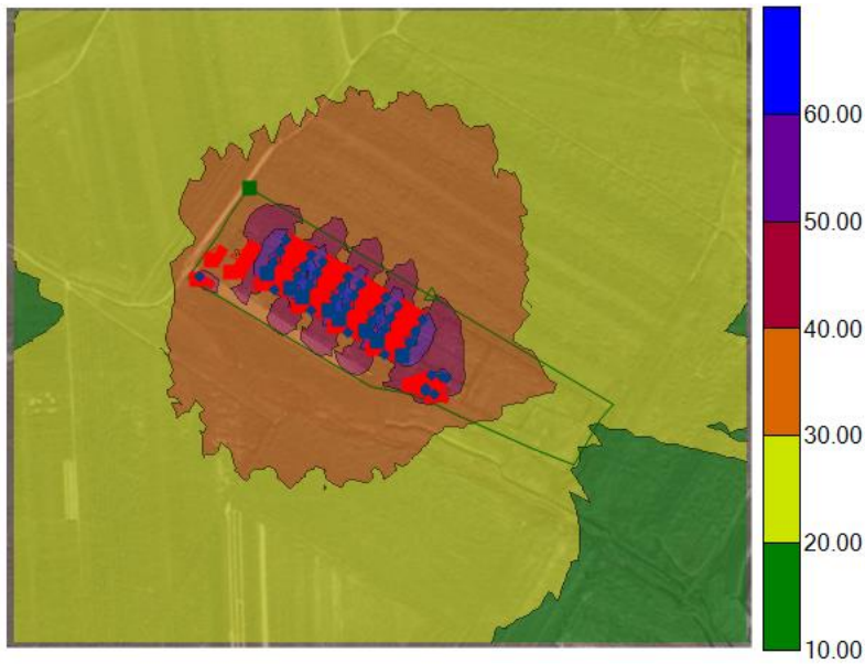
图 5.2-2 (a) 非采暖季噪声贡献值等值线分布图
