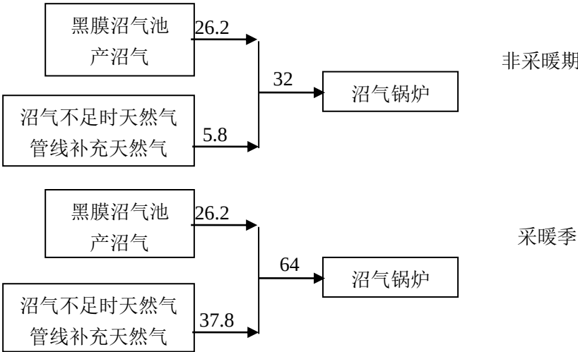
图 3.12-4 本项目沼气平衡图 单位：m 3 /d
