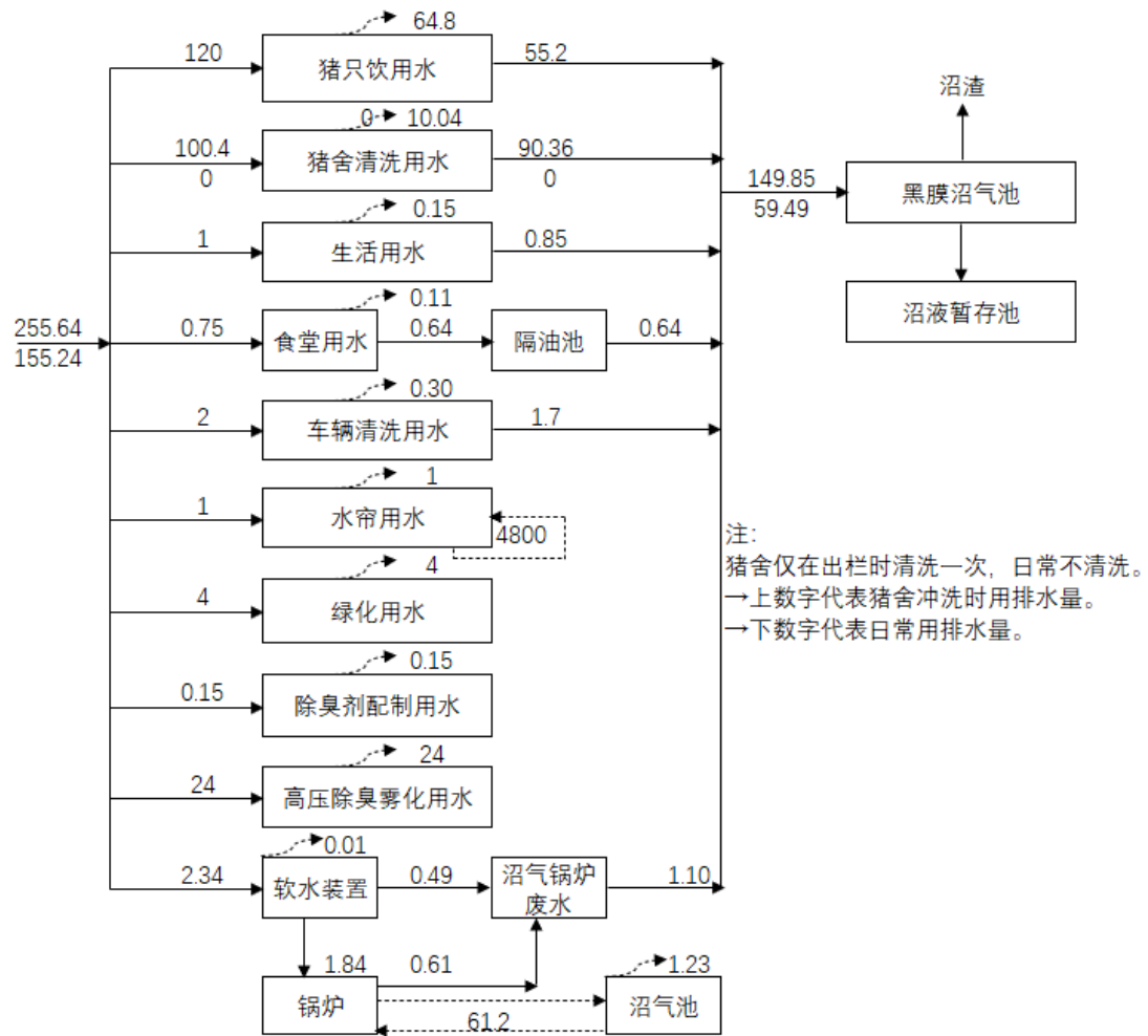
图 3.12-1 本项目夏季（120 天）水平衡图 单位：m³/d
