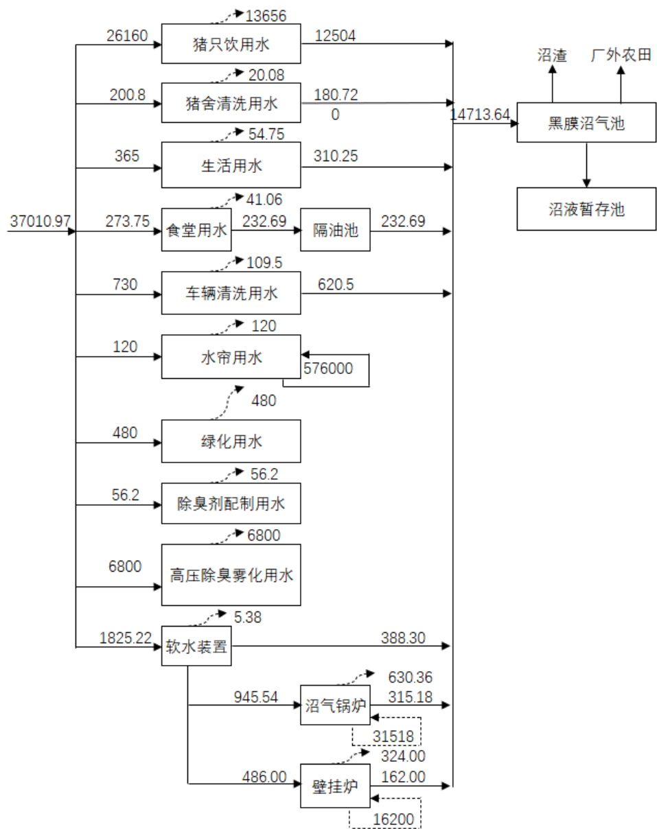
图 3.12-3 本项目水平衡图 单位：m³/a
