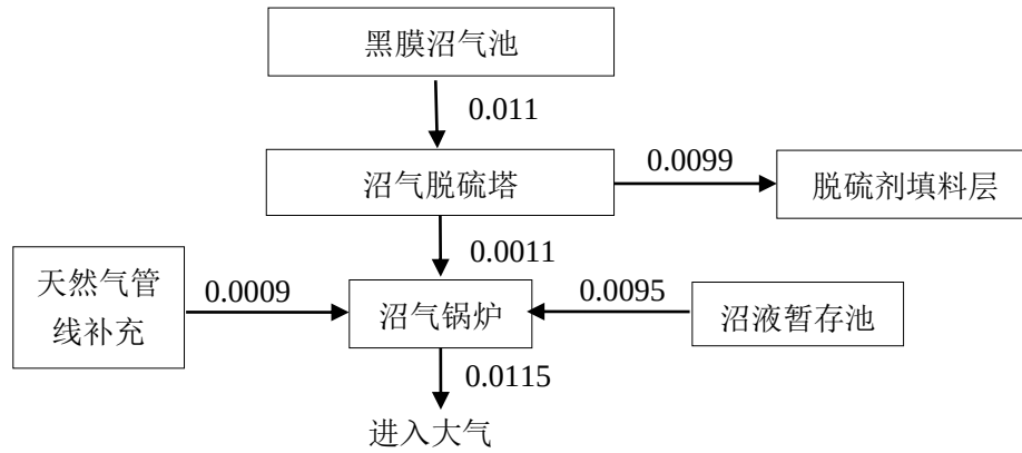
图 3.12-5 本项目沼气硫平衡图 单位：t/a
