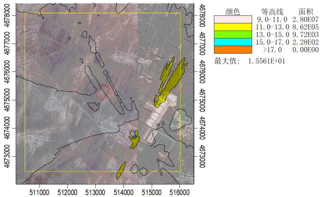
图 5.2-23 叠加现状浓度后 H 2 S 小时浓度贡献值分布图/ \mu\text{g}/\text{m}^3
