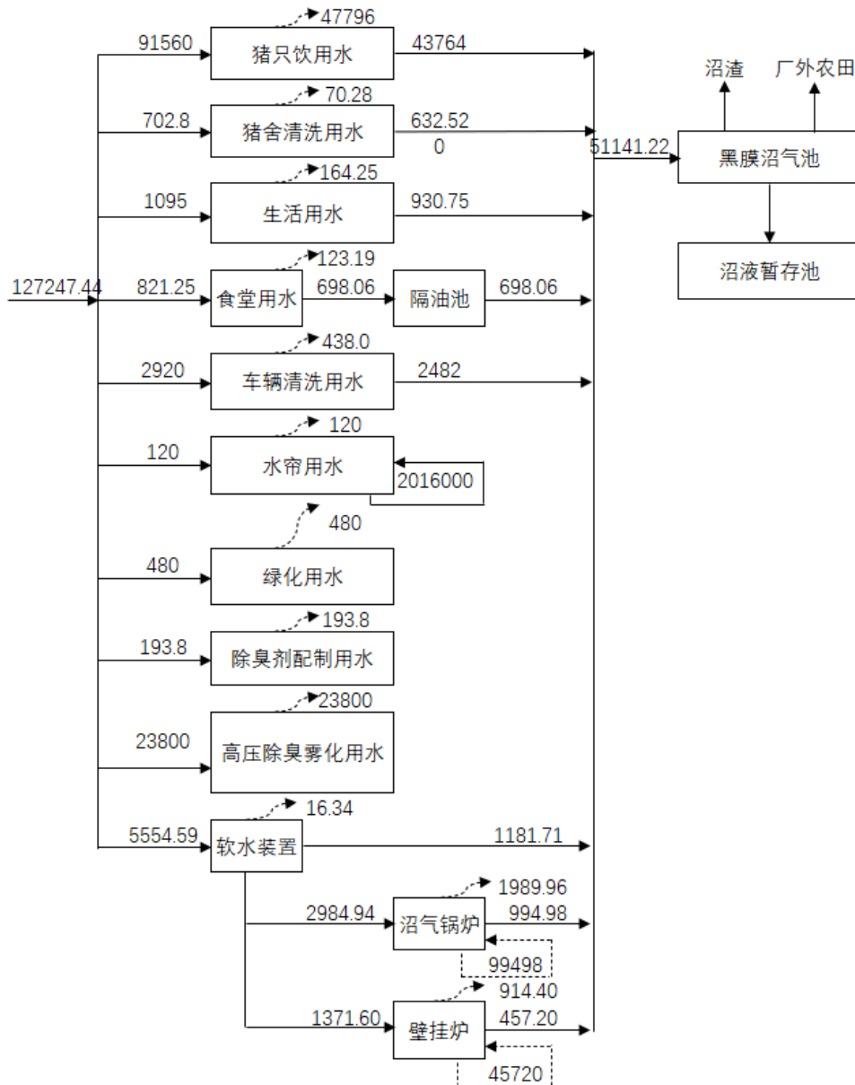
图 3.12-3 本项目水平衡图 单位: \text{m}^3/\text{a}
