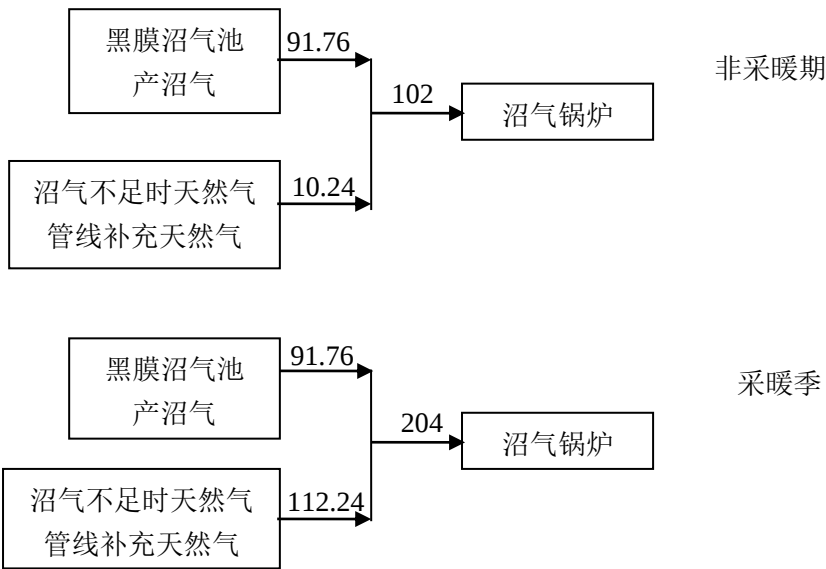
图 3.12-4 本项目沼气平衡图 单位：m 3 /d
