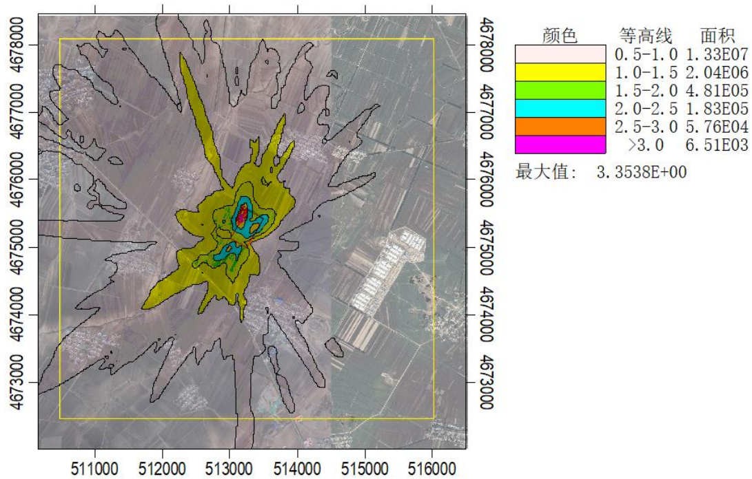
图 5.2-18 本项目 PM 10 日均浓度贡献值分布图/ \mu\text{g}/\text{m}^3
