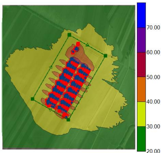
图 5.2-29 (a) 非采暖季噪声贡献值等值线分布图
