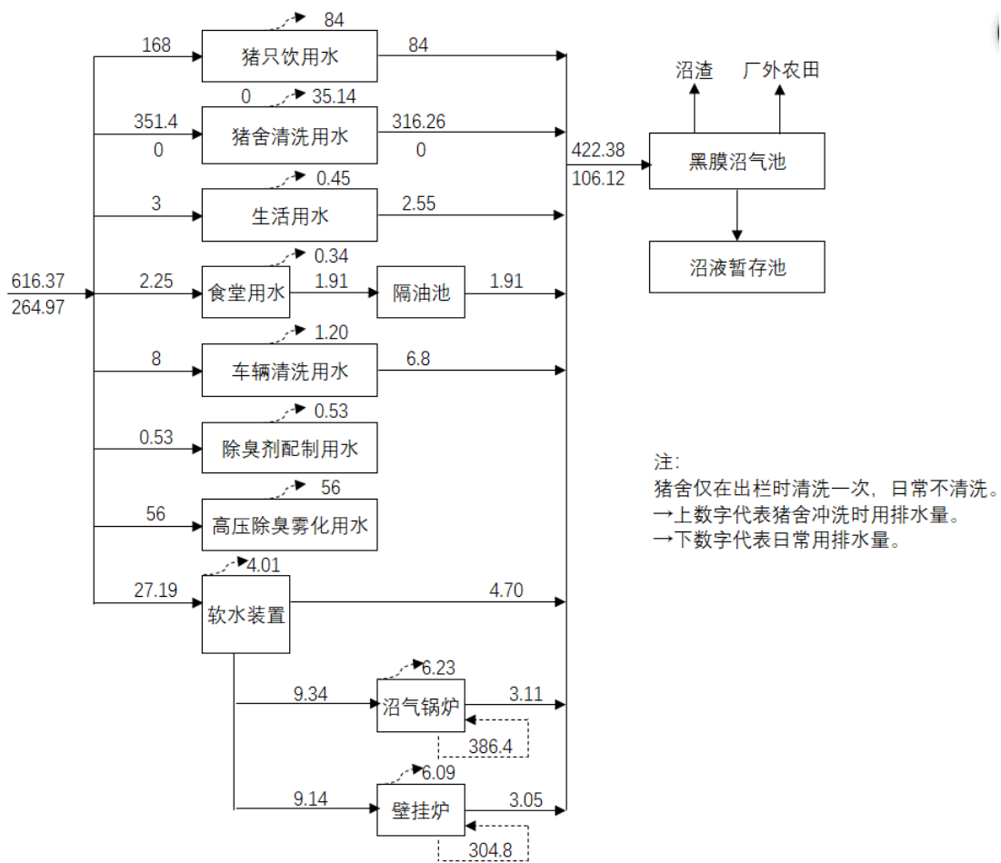
图 3.12-2 本项目其他季节（245 天）水平衡图 单位：m³/d
