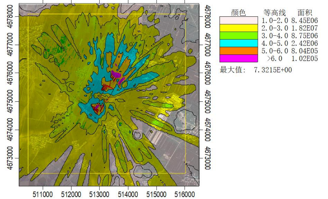
图 5.2-12 本项目二氧化硫小时浓度贡献值分布图/ \mu\text{g}/\text{m}^3
