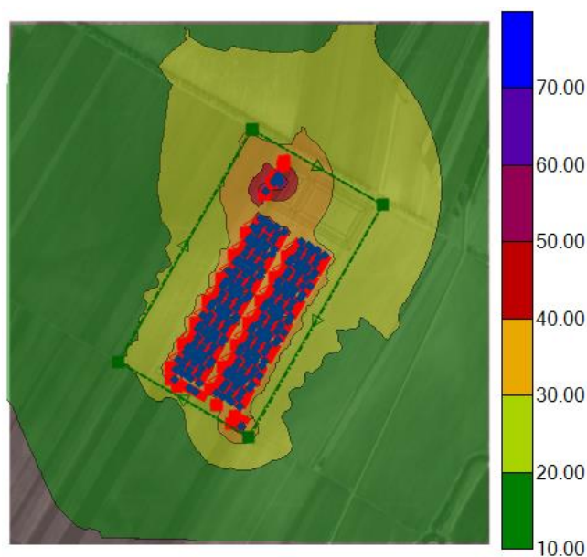
图 5.2-29 (b) 采暖季噪声贡献值等值线分布图
