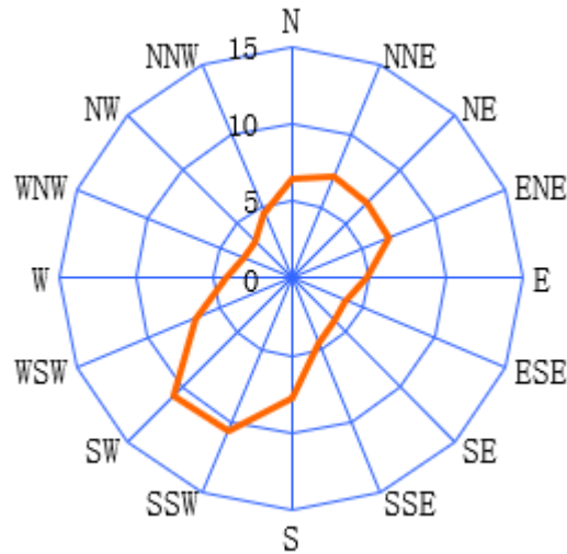
图 5.2-1 沈阳风向玫瑰图 (静风频率 4.28%)
