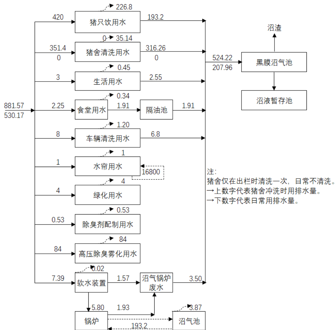
图 3.12-1 本项目夏季（120 天）水平衡图 单位：m³/d
