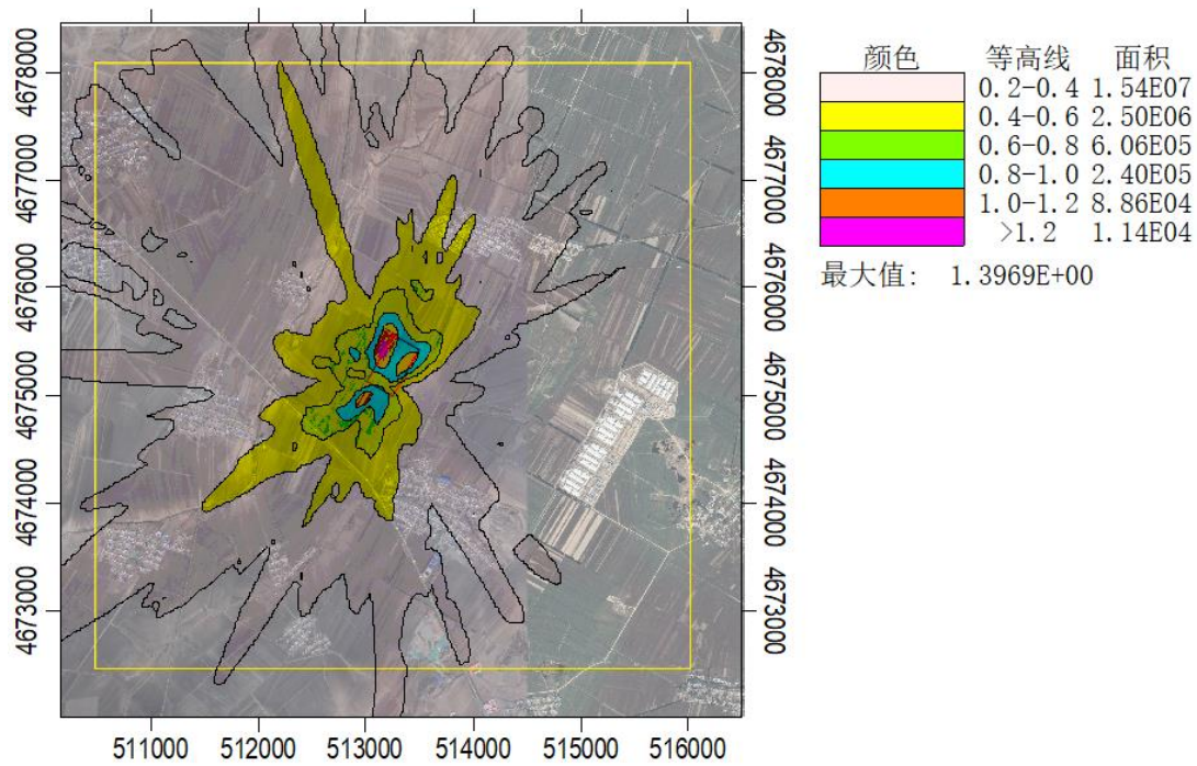
图 5.2-13 本项目二氧化硫日均浓度贡献值分布图/ \mu\text{g}/\text{m}^3
