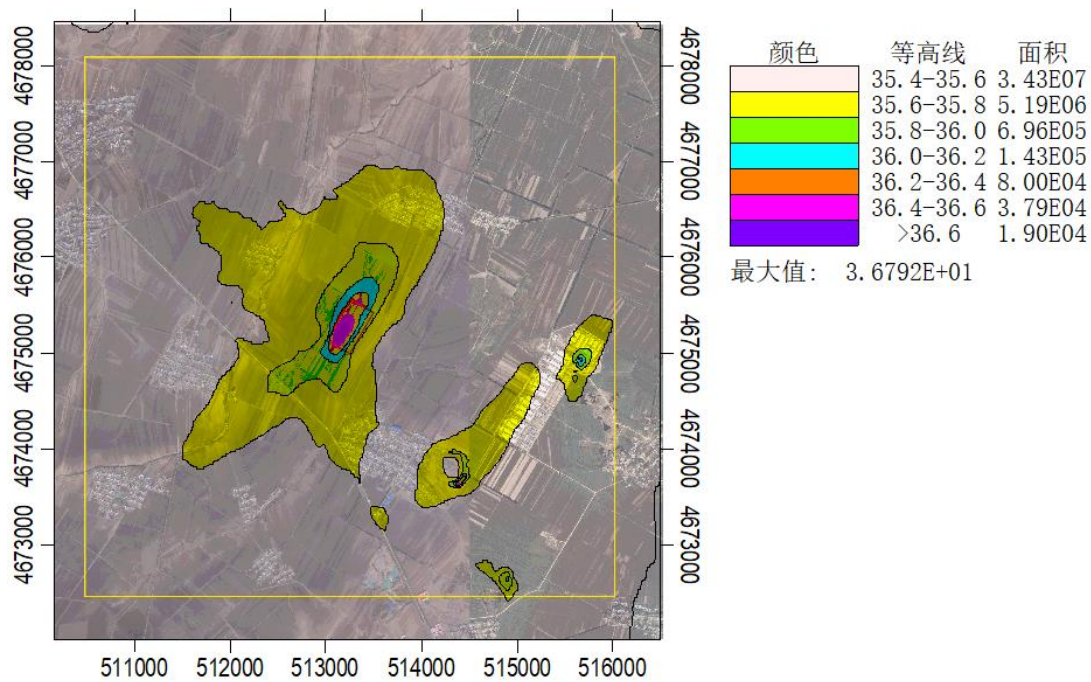
图 5.2-27 叠加现状浓度后 NOx 年均质量浓度分布图
