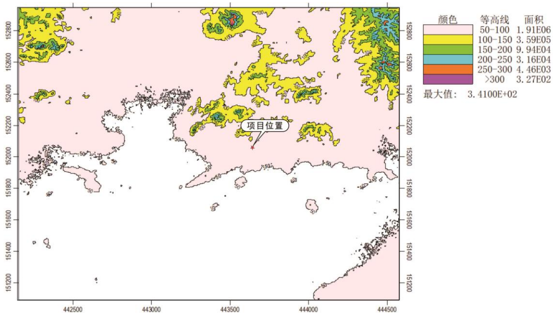
图 5.2-10 预测地形高程图
