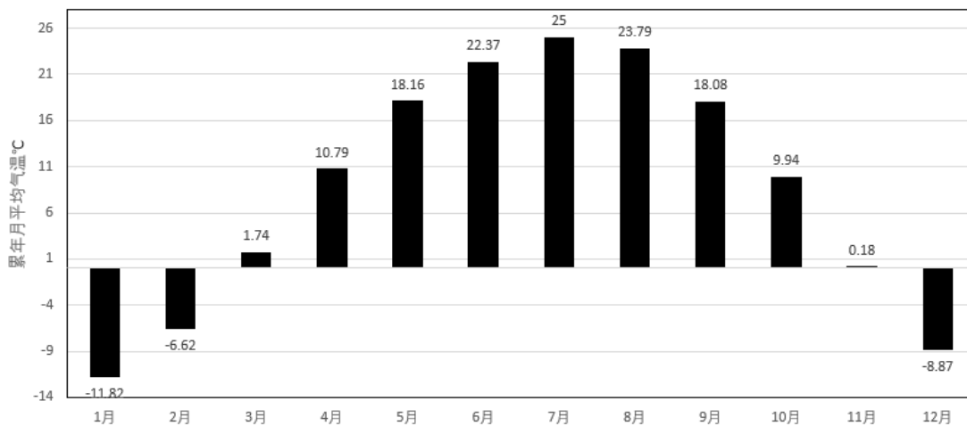
图 5.2-3 沈阳累年月平均气温（单位：℃）
