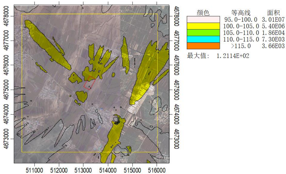
图 5.2-22 叠加现状浓度后 NH 3 小时浓度贡献值分布图/ \mu\text{g}/\text{m}^3
