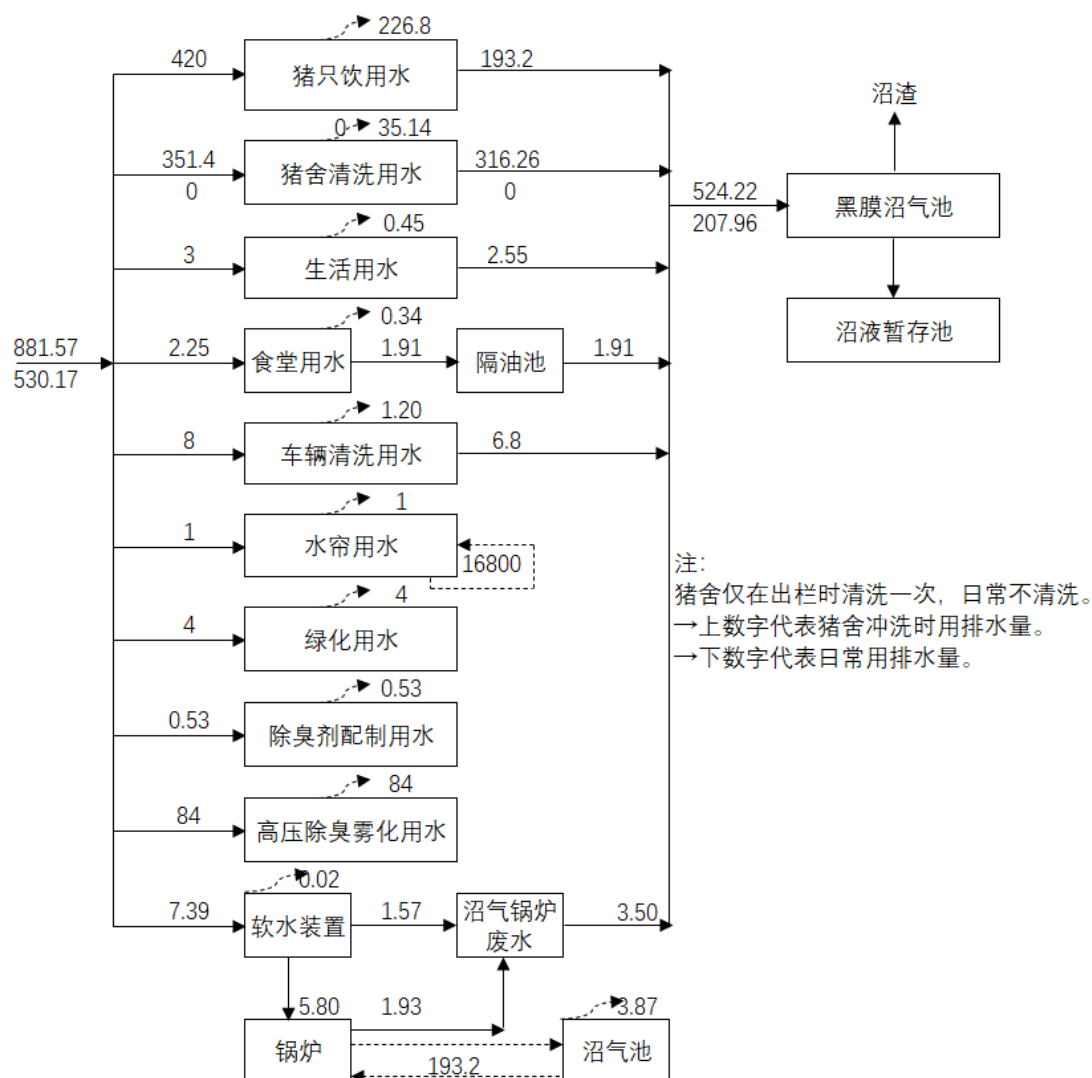
图 3.11-1 本项目夏季（120 天）水平衡图 单位：m³/d
