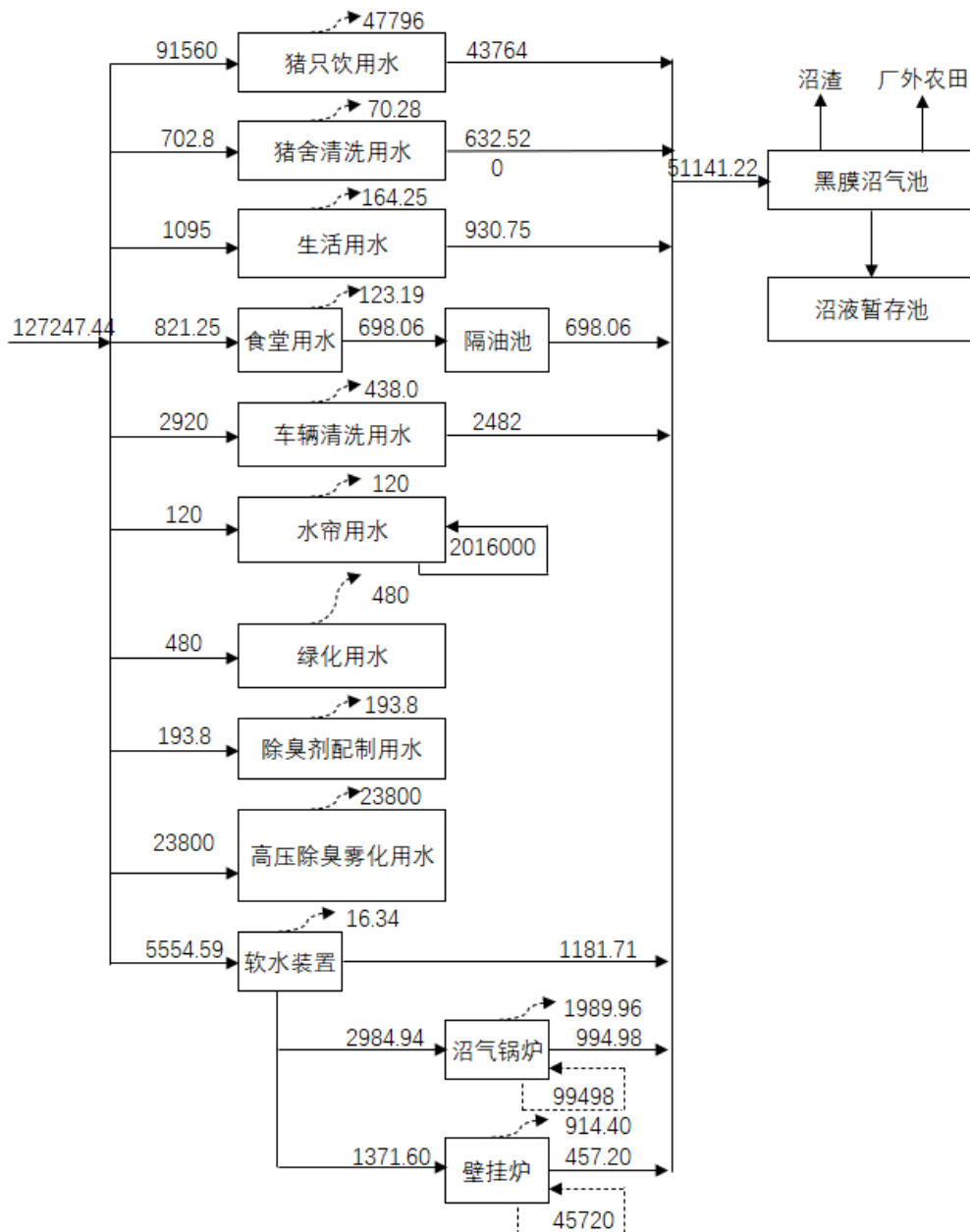
图 3.11-3 本项目水平衡图 单位: \text{m}^3/\text{a}
