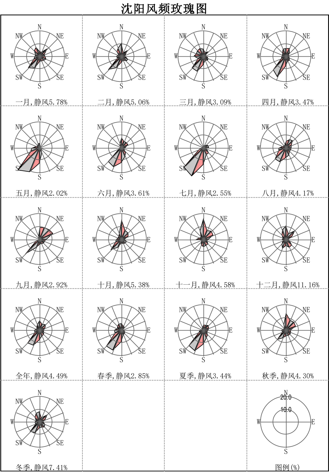
图 5.2-7 沈阳地区 2019 年及各月风玫瑰图
