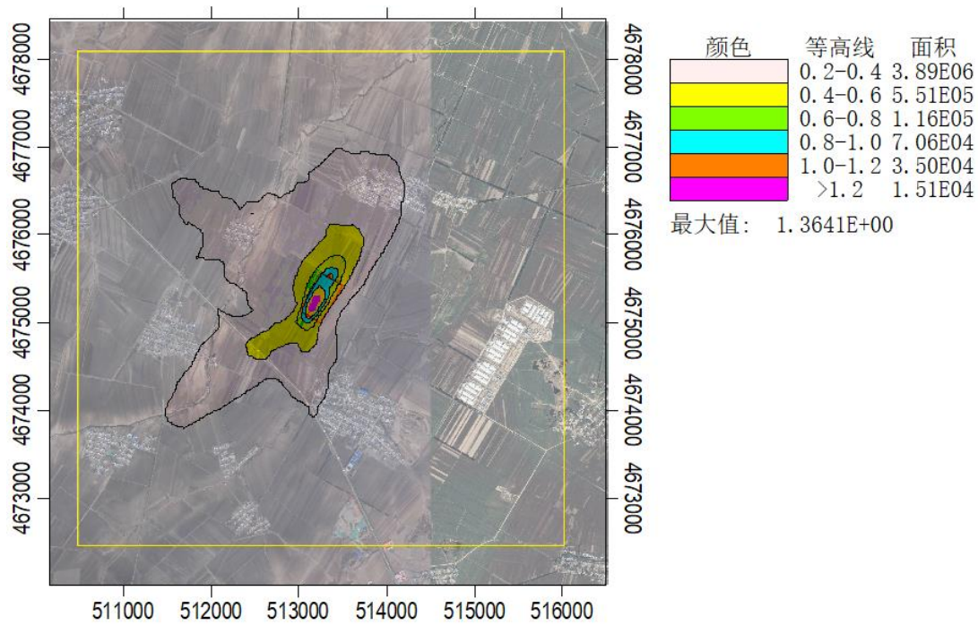
图 5.2-17 本项目氮氧化物年均浓度贡献值分布图/ \mu\text{g}/\text{m}^3
