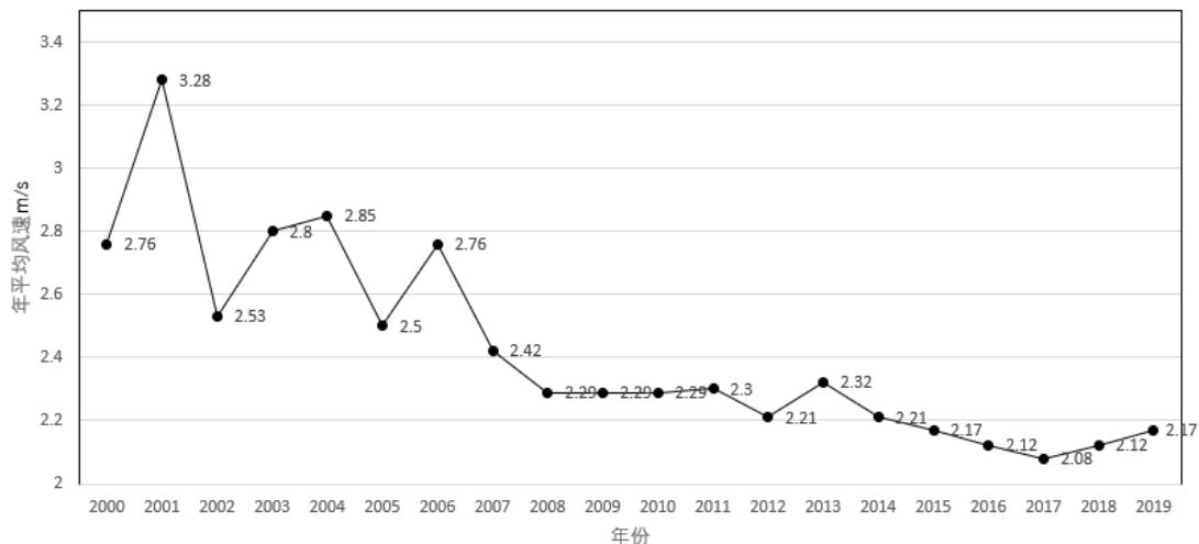
图 5.2-2 沈阳（2000-2019）年平均风速（单位：m/s）
