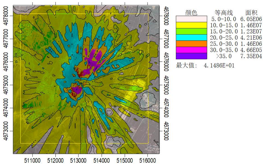
图 5.2-15 本项目氮氧化物小时浓度贡献值分布图/ \mu\text{g}/\text{m}^3
