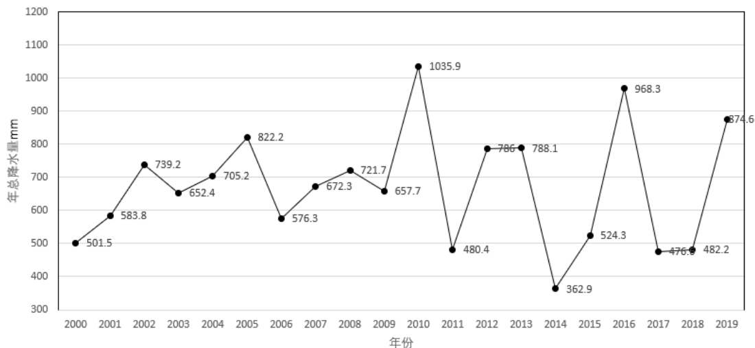
图 5.2-6 沈阳（2000-2019）年总降水量（单位：毫米）
