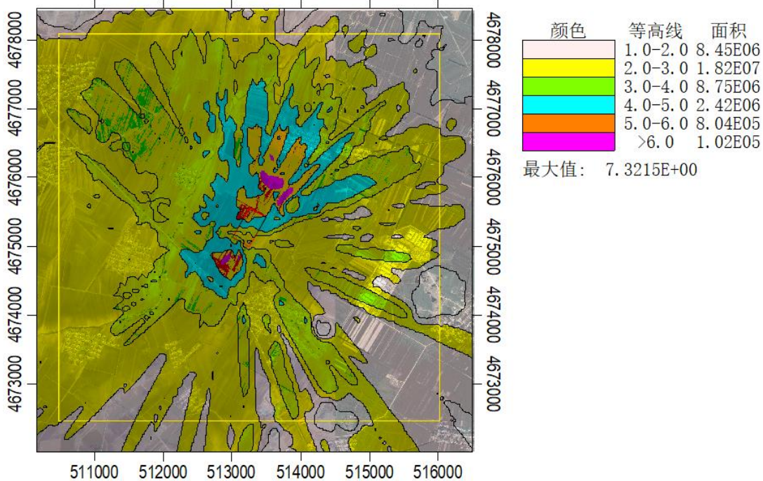
图 5.2-12 本项目二氧化硫小时浓度贡献值分布图/ \mu\text{g}/\text{m}^3
