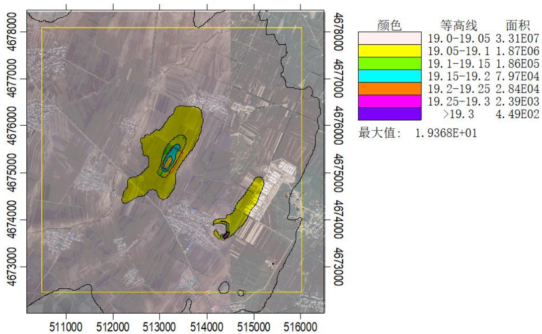
图 5.2-24 叠加现状浓度后 SO 2 年均质量浓度分布图
