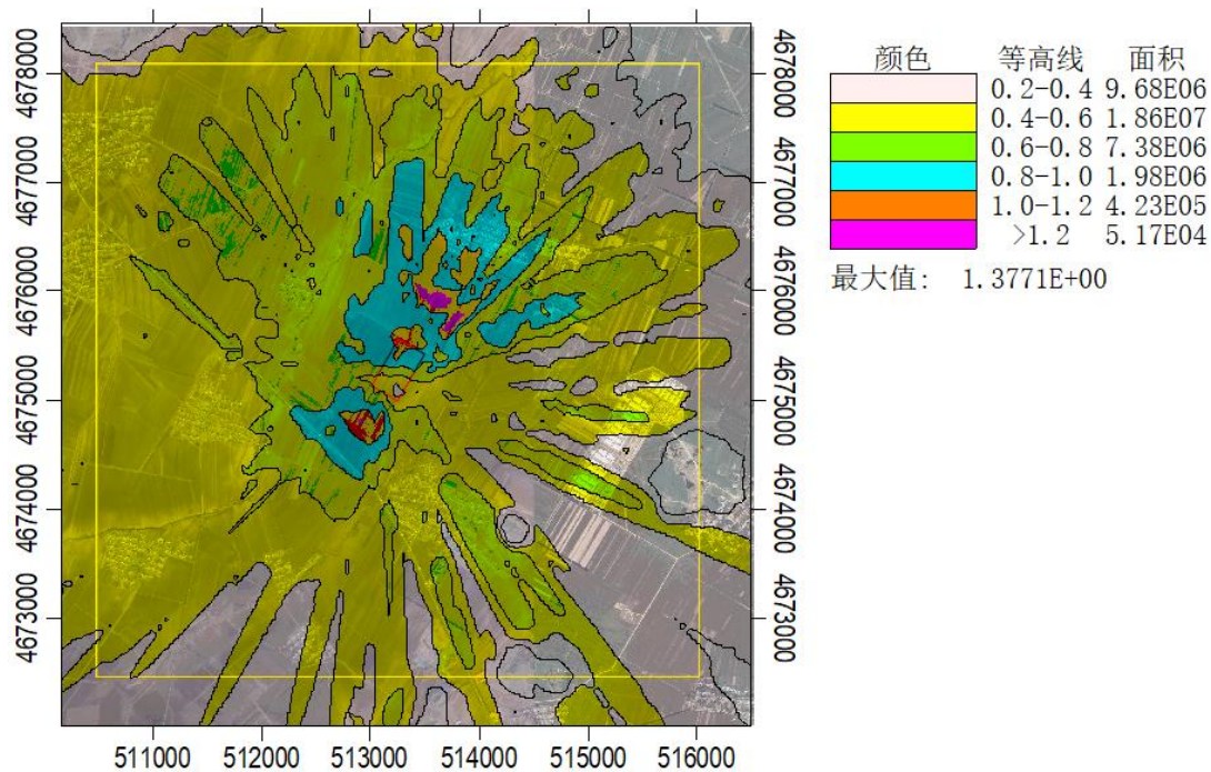
图 5.2-21 本项目 H 2 S 小时浓度贡献值分布图/µg/m 3
