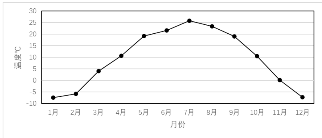
图 5.2-9 沈阳地区 2019 年平均温度月变化
