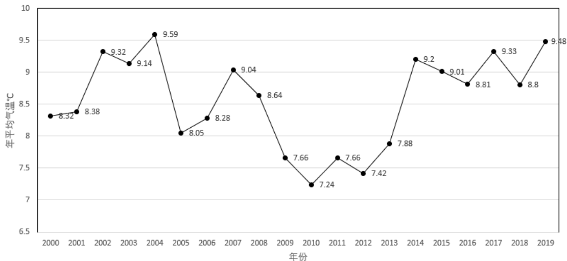
图 5.2-4 沈阳（2000-2019）年平均气温（单位：°C）
