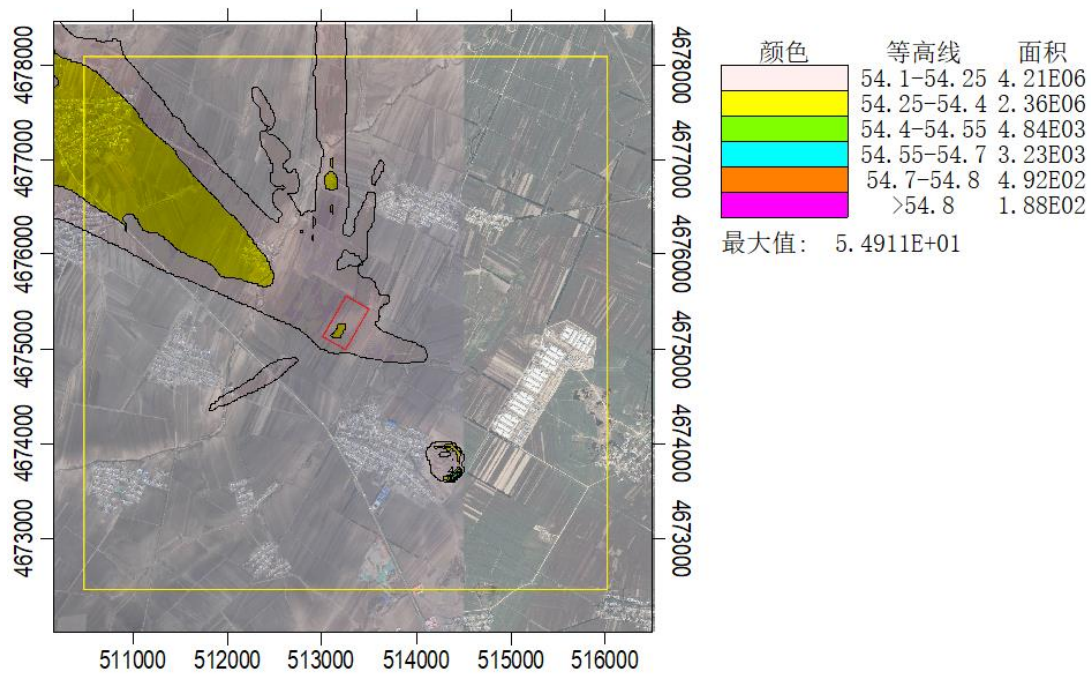
图 5.2-25 叠加现状浓度后 NO x 第 98 百分位保证率日平均质量浓度分布图
