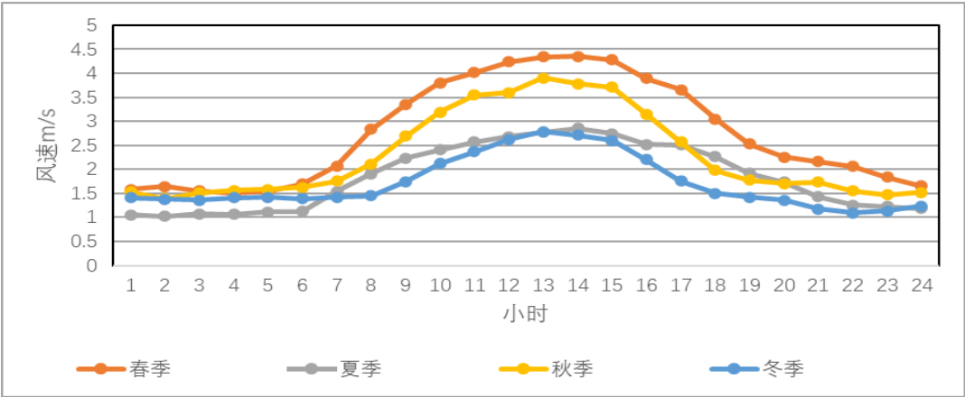
图 5.2-8 沈阳地区 2019 年季小时平均风速日变化
