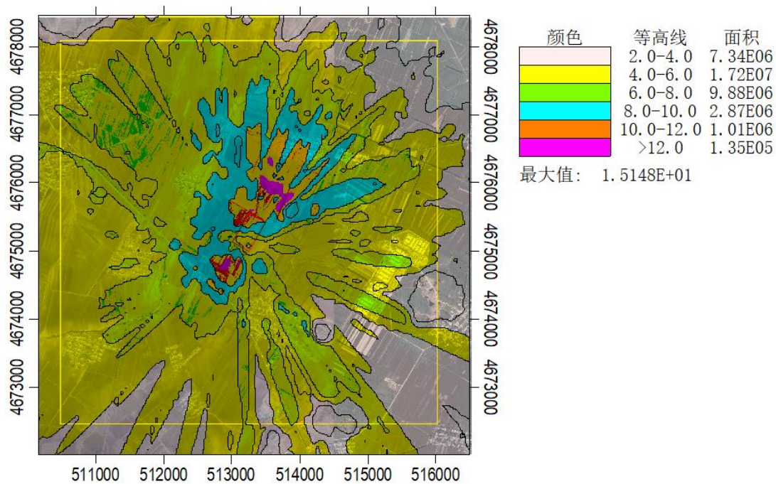
图 5.2-20 本项目 NH 3 小时浓度贡献值分布图/ \mu\text{g}/\text{m}^3
