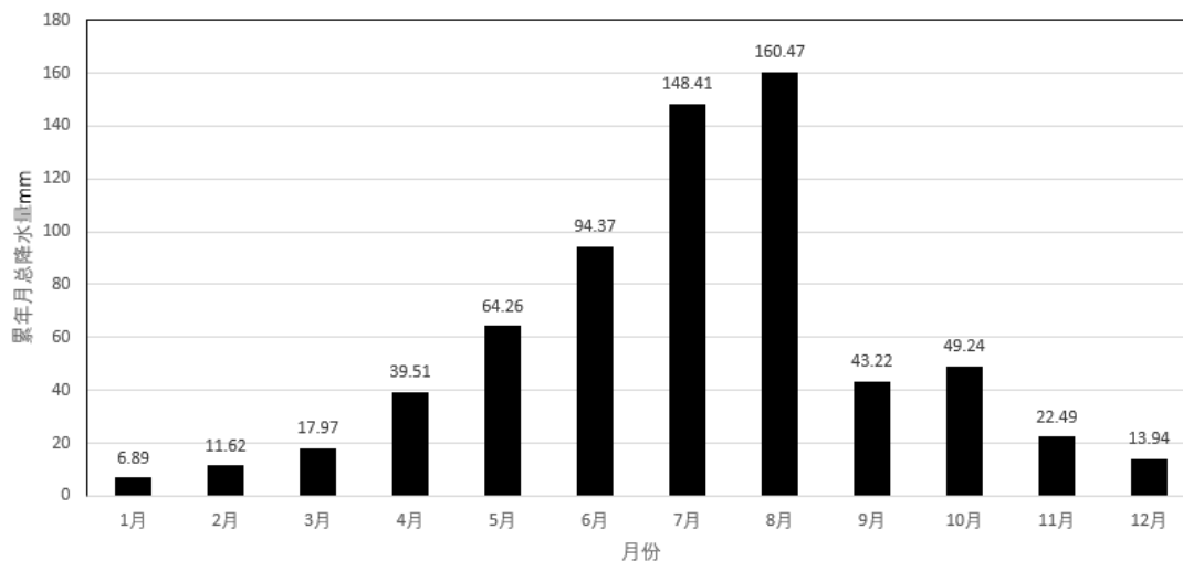
图 5.2-5 沈阳月平均降水量（单位：mm）
