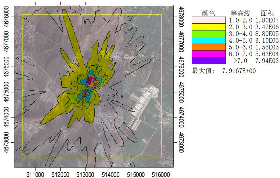
图 5.2-16 本项目氮氧化物日均浓度贡献值分布图/ \mu\text{g}/\text{m}^3
