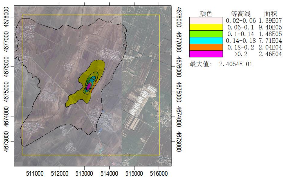
图 5.2-14 本项目二氧化硫年均浓度贡献值分布图/ \mu\text{g}/\text{m}^3
