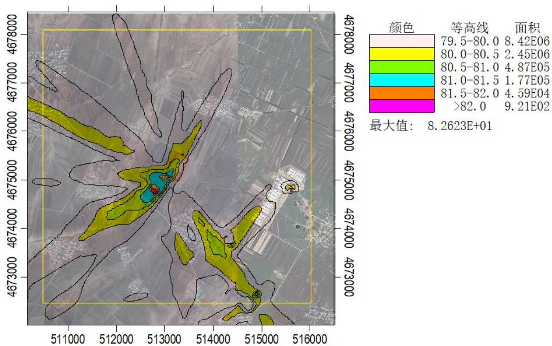
图 5.2-26 叠加现状浓度后 NO x 第 98 百分位保证率日平均质量浓度分布图
