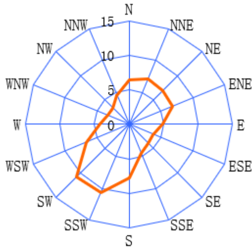
图 5.2-1 沈阳风向玫瑰图（静风频率 4.28%）
