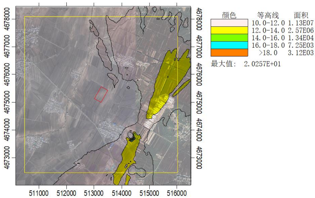
图 5.2-23 叠加现状浓度后 H 2 S 小时浓度贡献值分布图/ \mu\text{g}/\text{m}^3
