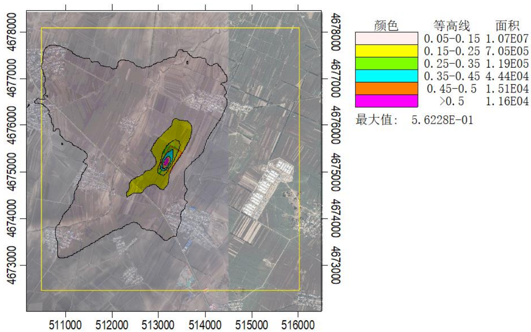
图 5.2-19 本项目 PM 10 年均浓度贡献值分布图/ \mu\text{g}/\text{m}^3
