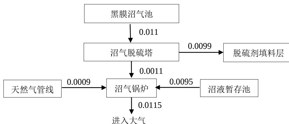
图 3.11-5 本项目沼气硫平衡图
