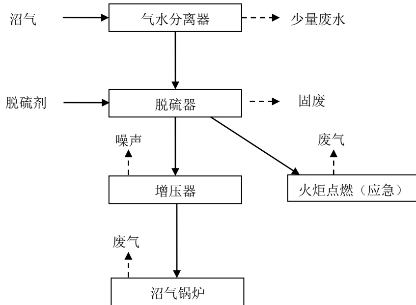
图 3.4-3 本项目沼气净化及综合利用工艺流程及产污节点图
