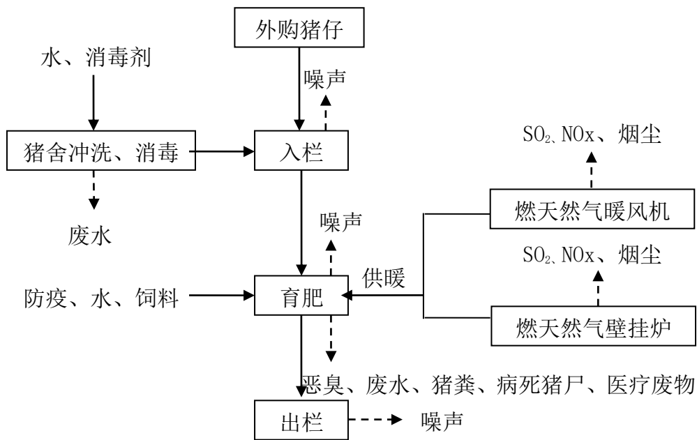
图 3.1-1 本项目养殖工艺流程及产污节点图
