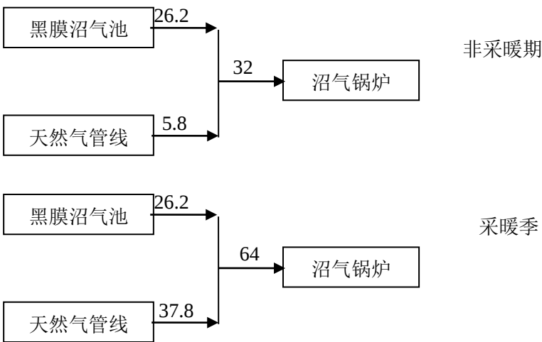
图 3.11-4 本项目沼气平衡图
