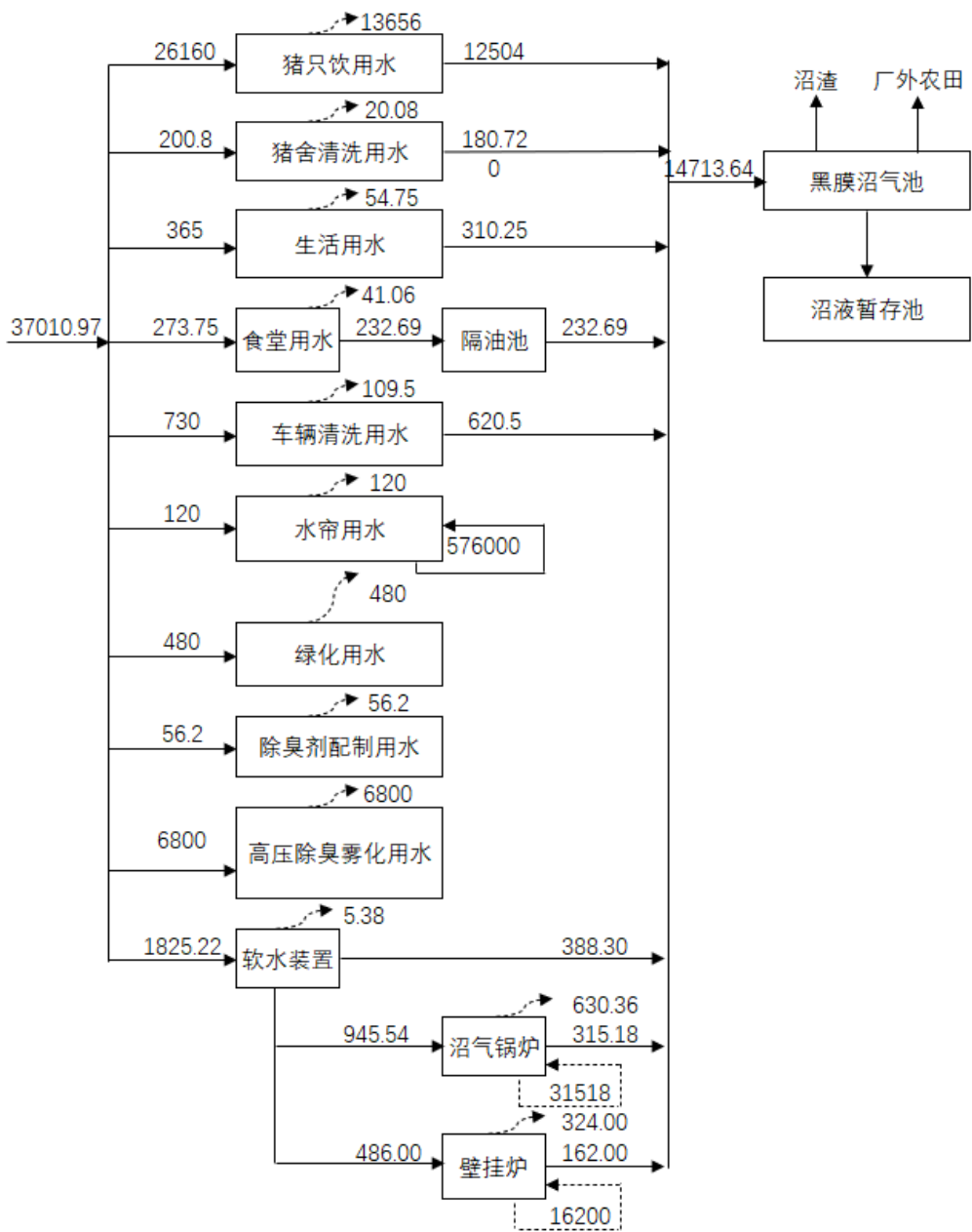
图 3.11-3 本项目水平衡图 单位: m³/a
