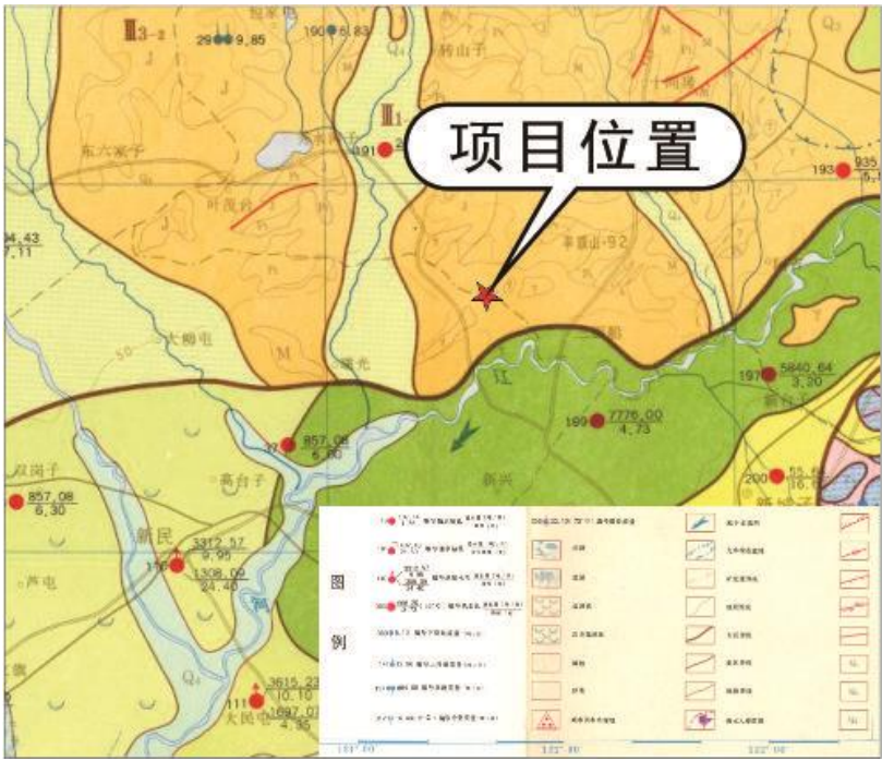
图 5.2-2 区域水文地质图部分截图（1:500000）
