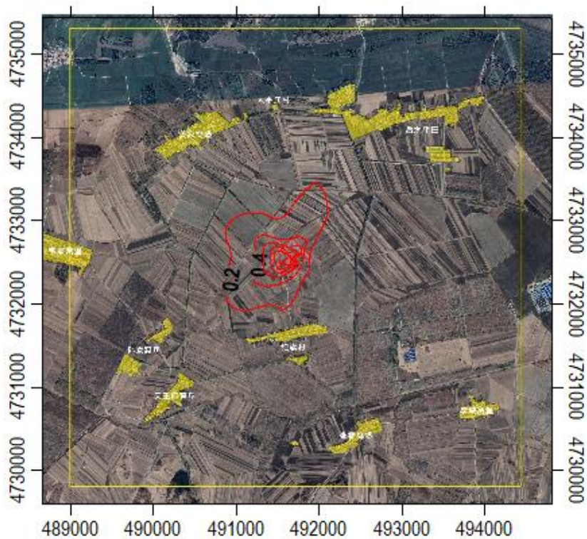
图 5.2-15 本项目氮氧化物年均浓度贡献值分布图/ \mu\text{g}/\text{m}^3
