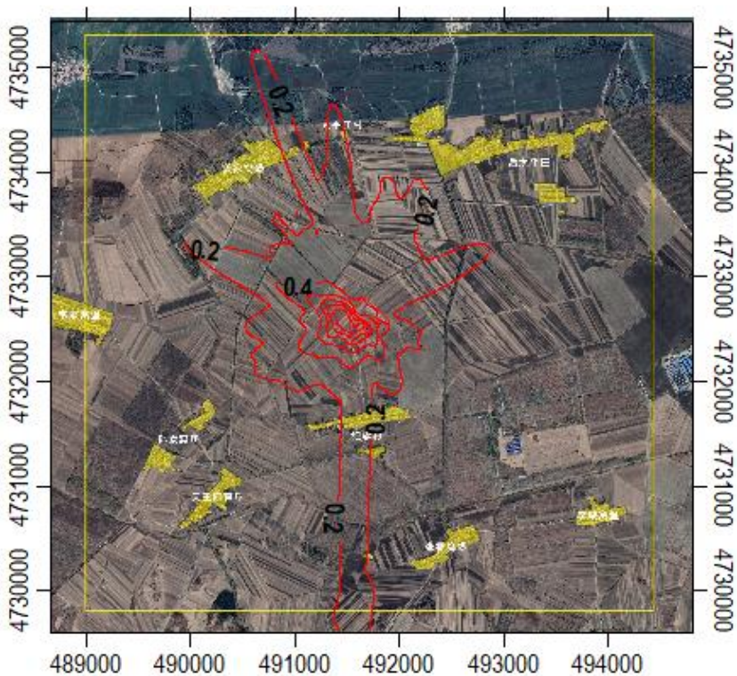
图 5.2-16 本项目 \text{PM}_{10} 日均浓度贡献值分布图/ \mu\text{g}/\text{m}^3
