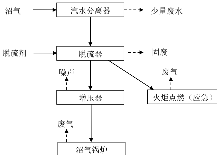
图 3.4-3 本项目沼气净化及综合利用工艺流程及产污节点图
