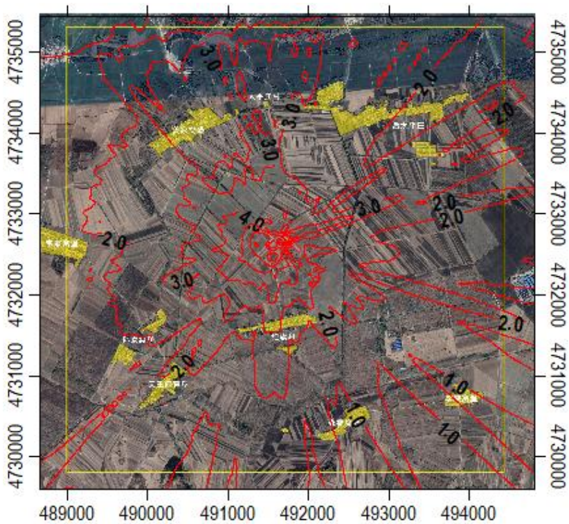
图 5.2-18 本项目 \text{NH}_3 小时浓度贡献值分布图/ \mu\text{g}/\text{m}^3
