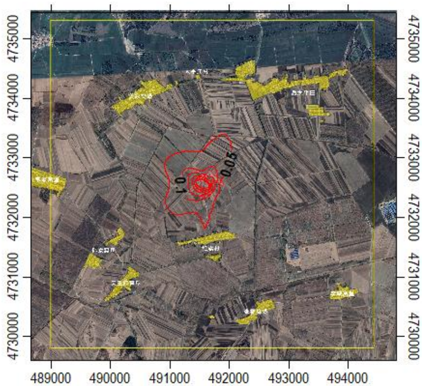
图 5.2-16 本项目 \text{PM}_{10} 年均浓度贡献值分布图/ \mu\text{g}/\text{m}^3
