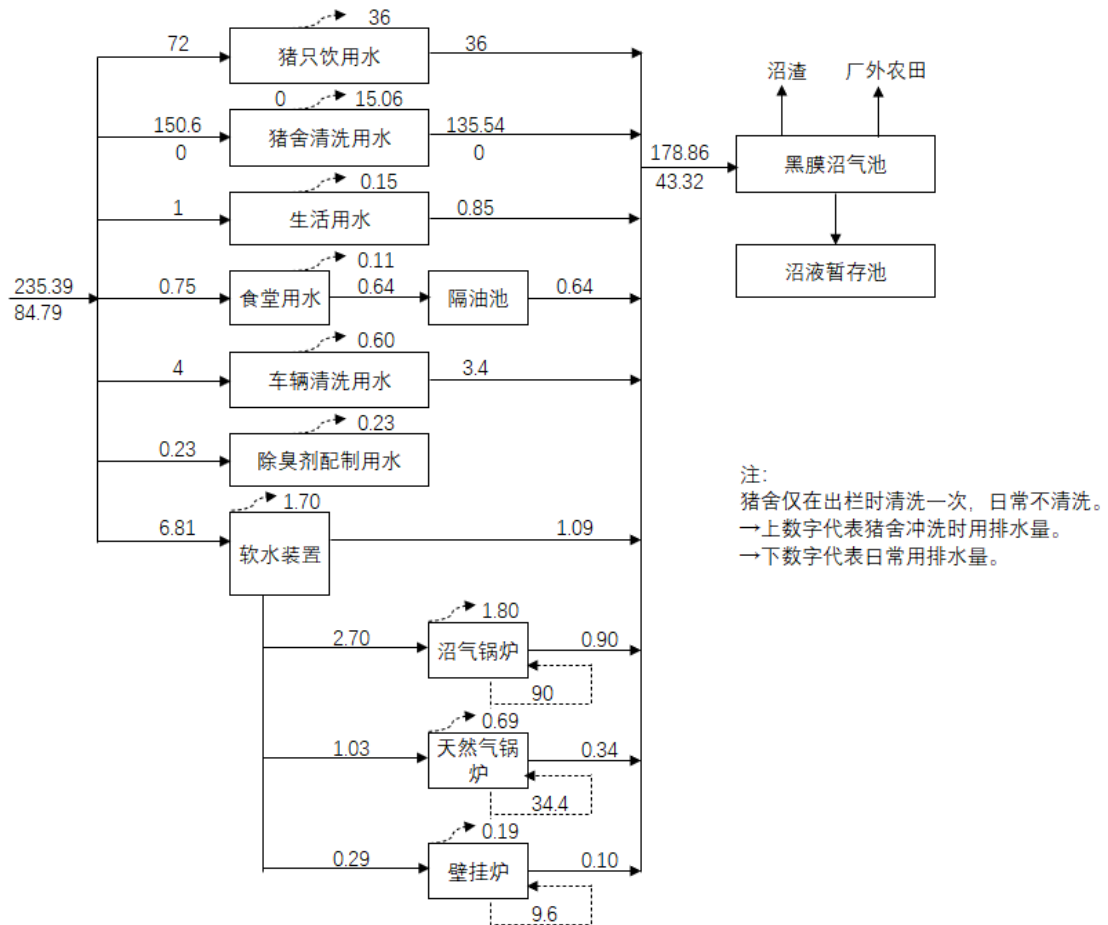
图 3.12-2 本项目其他季节（245 天）水平衡图 单位：m 3 /d
