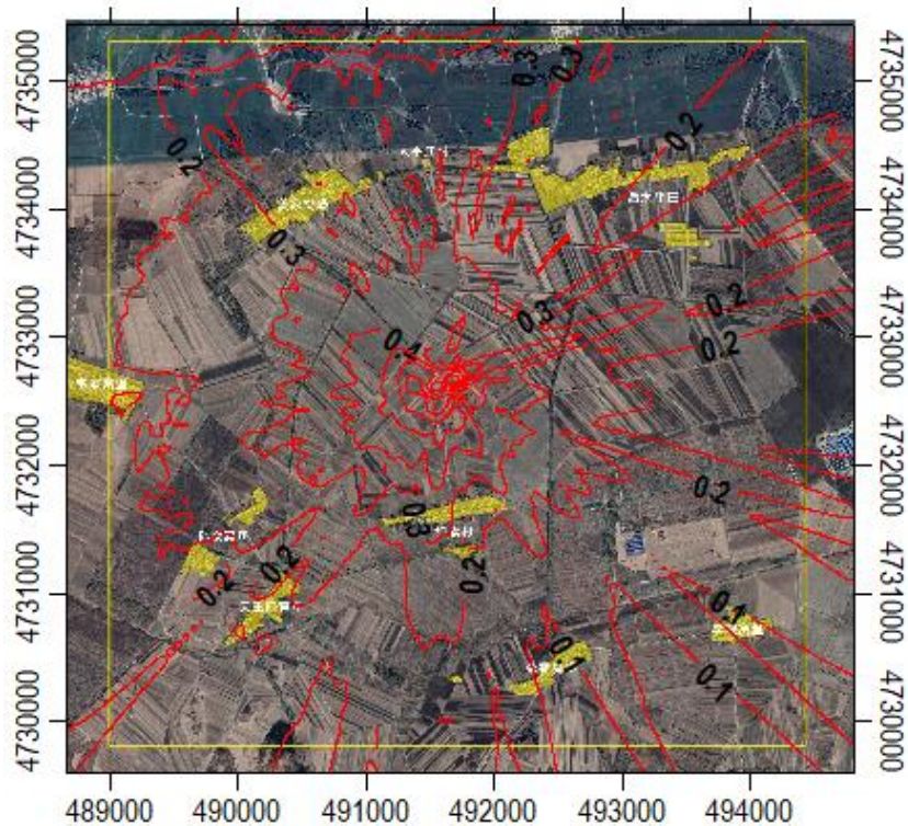
图 5.2-19 本项目 H 2 S 小时浓度贡献值分布图/μg/m 3
