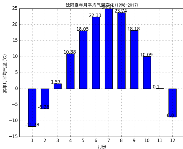
图 5.2-3 沈阳月平均气温 (单位: °C)
