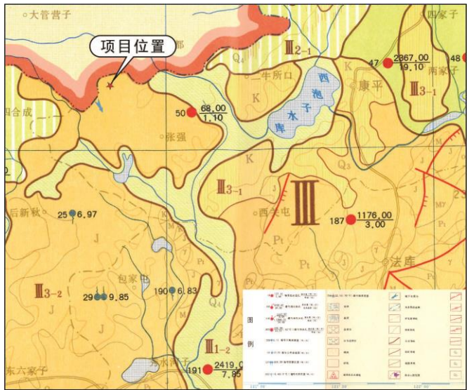
图 5.2-3 区域水文地质图部分截图（1:500000）
