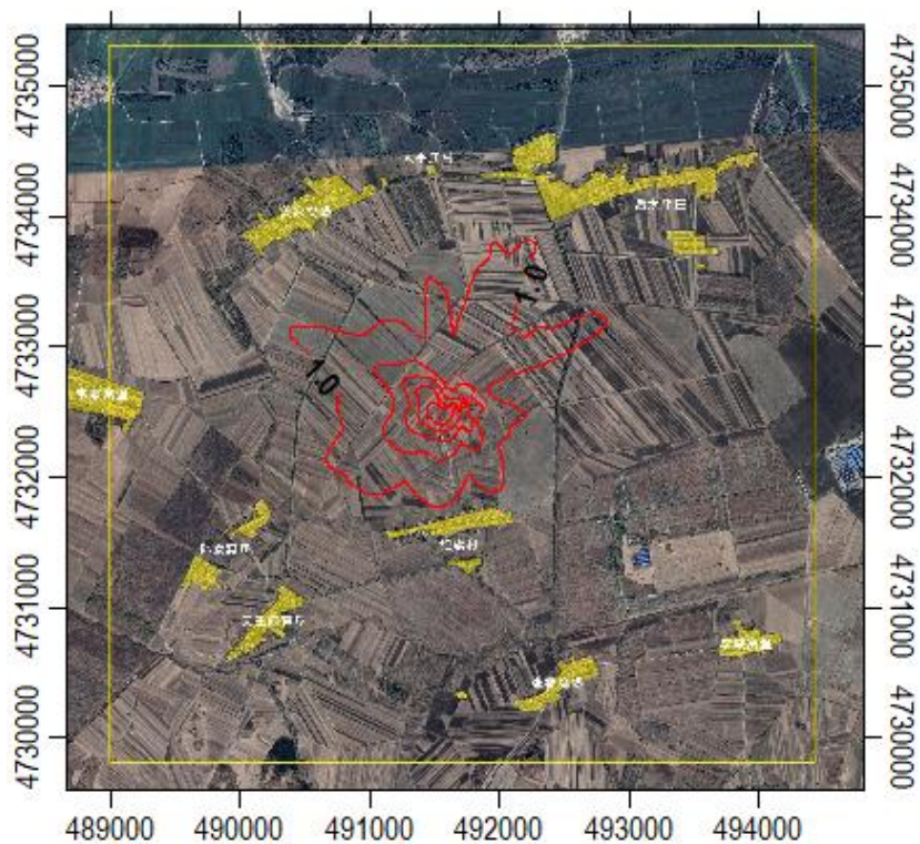
图 5.2-14 本项目氮氧化物日均浓度贡献值分布图/ \mu\text{g}/\text{m}^3
