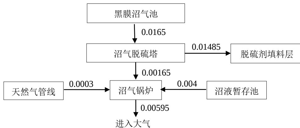
图 3.12-5 本项目沼气硫平衡图
