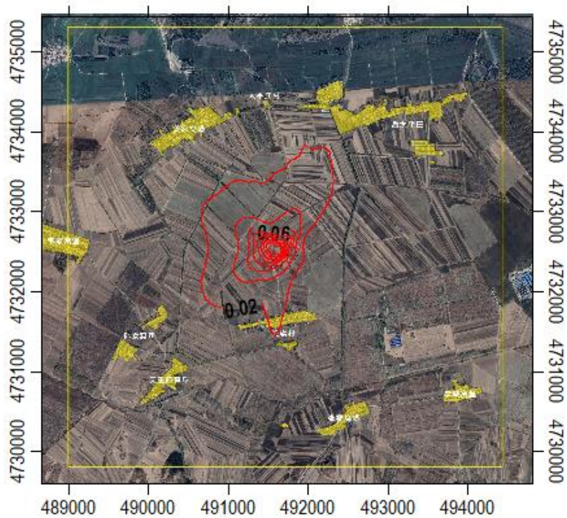
图 5.2-12 本项目二氧化硫年均浓度贡献值分布图/ \mu\text{g}/\text{m}^3
