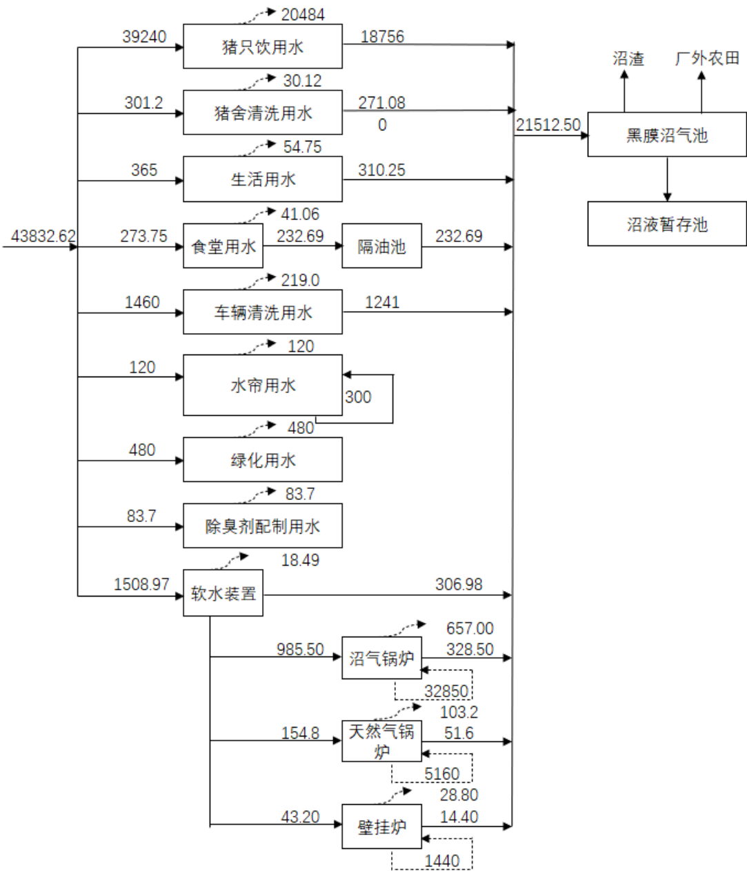
图 3.12-3 本项目水平衡图 单位：m³/a
