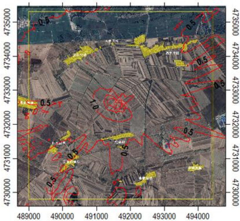
图 5.2-10 本项目二氧化硫小时浓度贡献值分布图/μg/m 3
