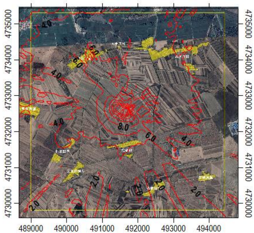
图 5.2-13 本项目氮氧化物小时浓度贡献值分布图/ \mu\text{g}/\text{m}^3
