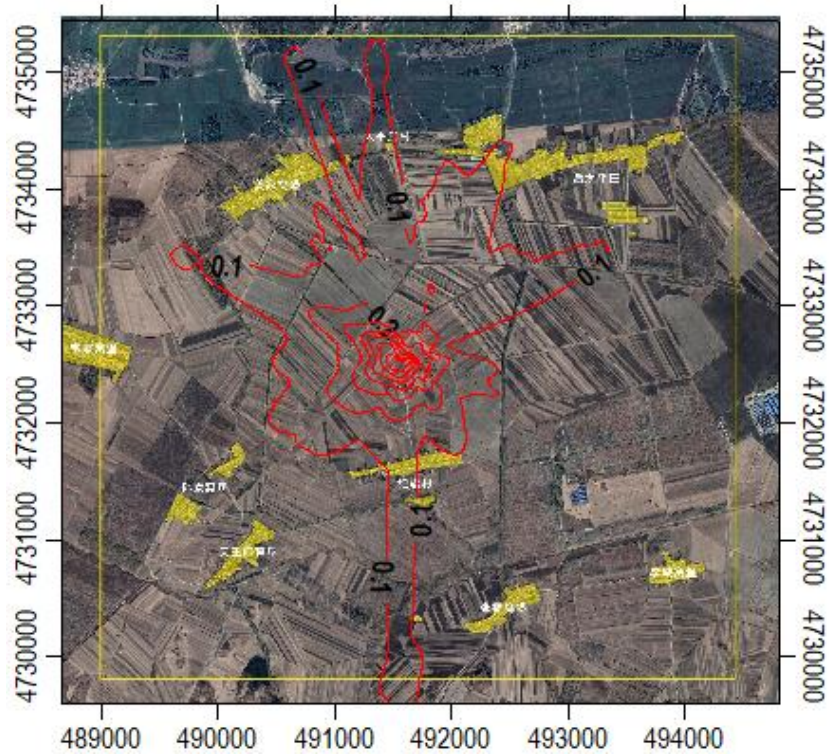
图 5.2-11 本项目二氧化硫日均浓度贡献值分布图/ \mu\text{g}/\text{m}^3
