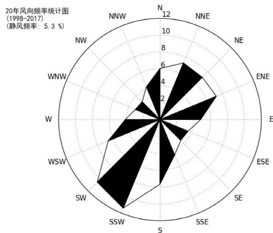
图 5.2-1 沈阳风向玫瑰图（静风频率 5.3%）
