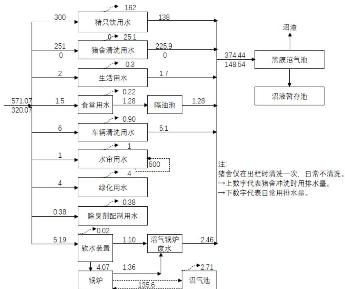
图 3.12-1 本项目夏季（120 天）水平衡图 单位：m³/d
