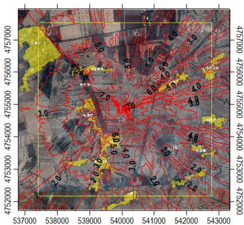
图 5.2-18 本项目 NH_3 小时浓度贡献值分布图/ \mu g/m^3
