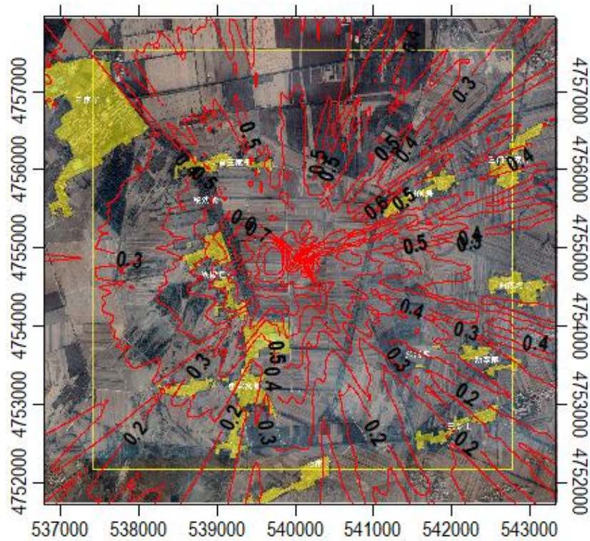
图 5.2-19 本项目 H 2 S 小时浓度贡献值分布图/µg/m 3
