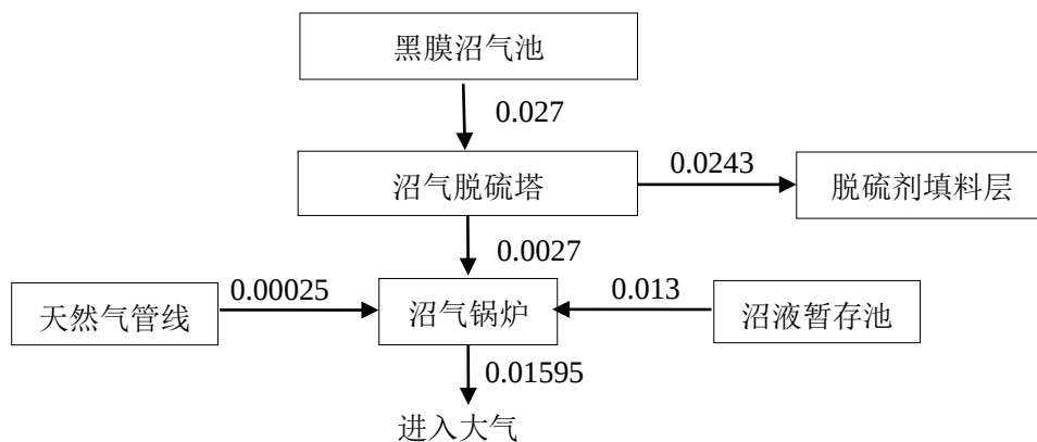
图 3.12-5 本项目沼气锅炉硫平衡图
