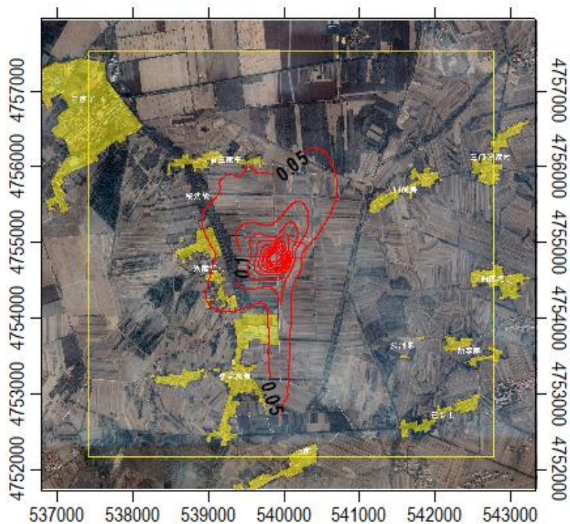
图 5.2-17 本项目 PM_{10} 年均浓度贡献值分布图/ \mu g/m^3
