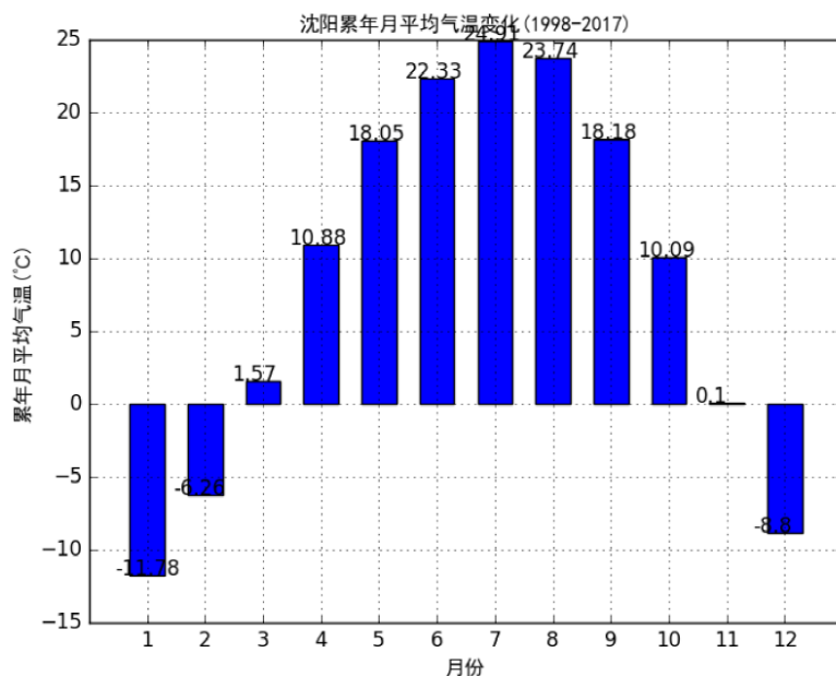
图 5.2-3 沈阳月平均气温（单位：℃）
