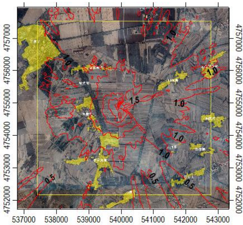
图 5.2-10 本项目二氧化硫小时浓度贡献值分布图/µg/m³
