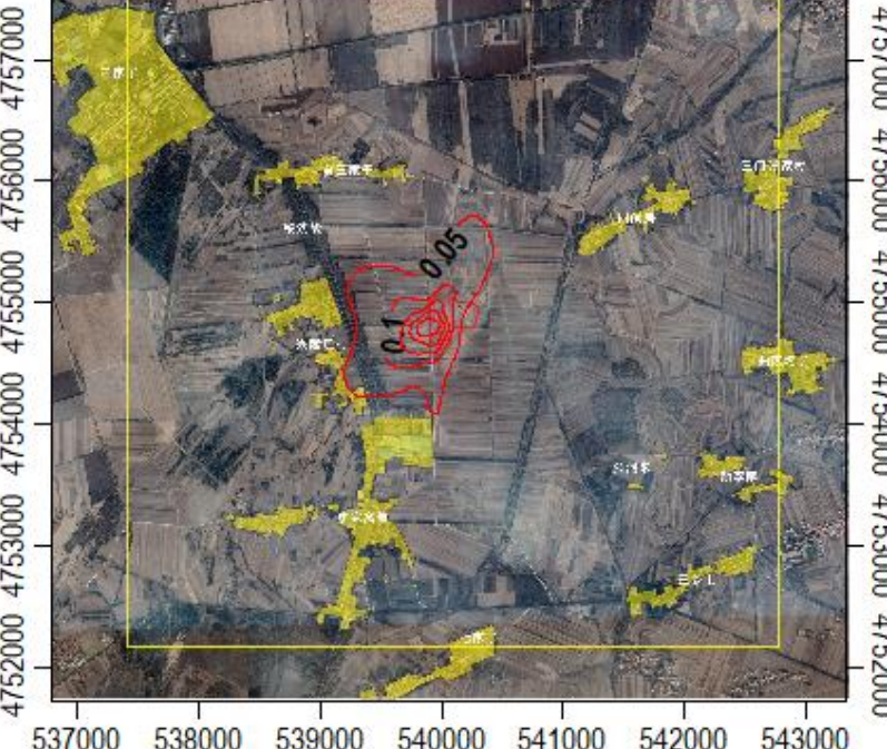
图 5.2-12 本项目二氧化硫年均浓度贡献值分布图/ \mu\text{g}/\text{m}^3
