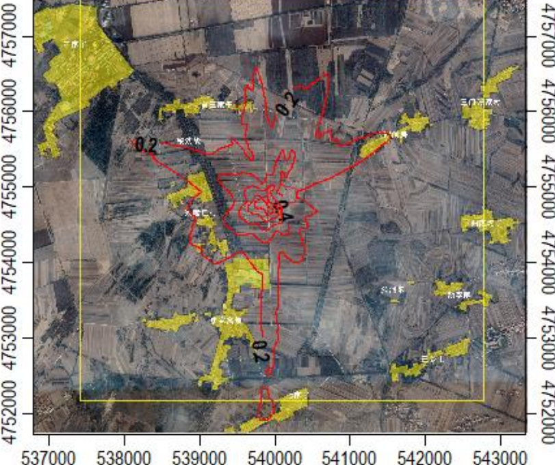
图 5.2-11 本项目二氧化硫日均浓度贡献值分布图/ \mu\text{g}/\text{m}^3
