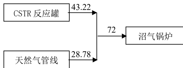
图 3.12-4 本项目沼气平衡图 单位：m 3 /d
