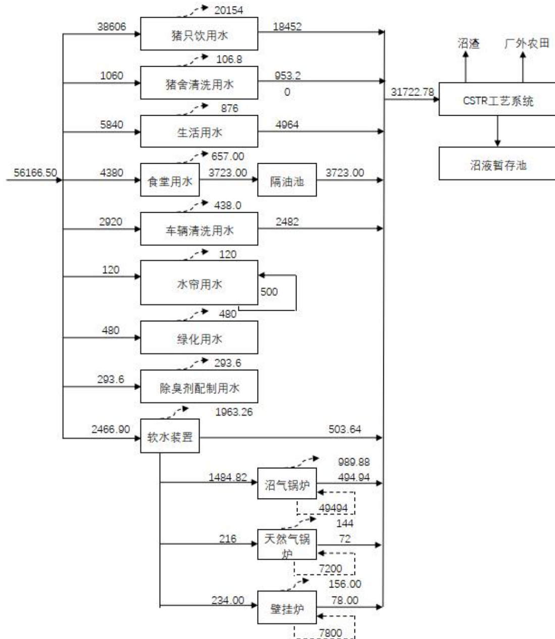
图 3.12-3 本项目水平衡图 单位：m³/a
