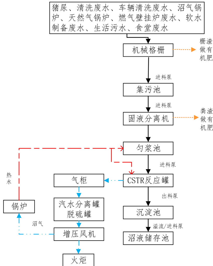
图 3.3-1 本项目粪污水处理工艺示意图
