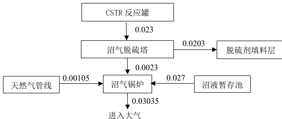
图 3.12-5 本项目沼气锅炉硫平衡图 单位：t
