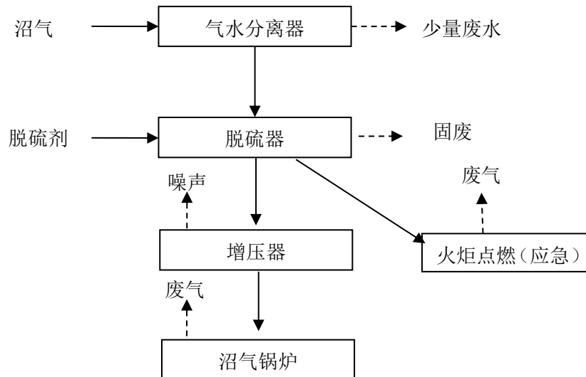
图 3.4-3 本项目沼气净化及综合利用工艺流程及产污节点图
