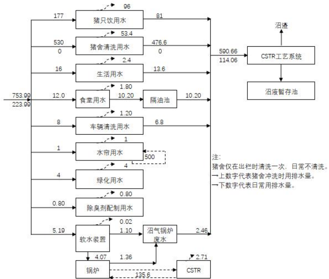
图 3.12-1 本项目夏季（120 天）水平衡图 单位：m³/d
