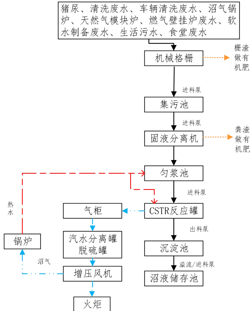
图 3.3-1 本项目粪污水处理工艺示意图
