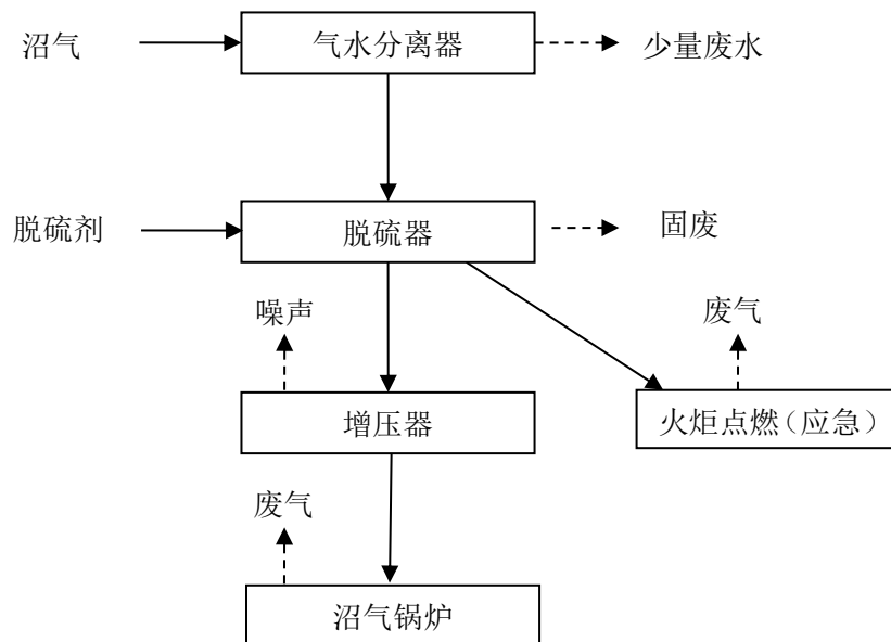
图 3.4-2 本项目沼气净化及综合利用工艺流程及产污节点图
