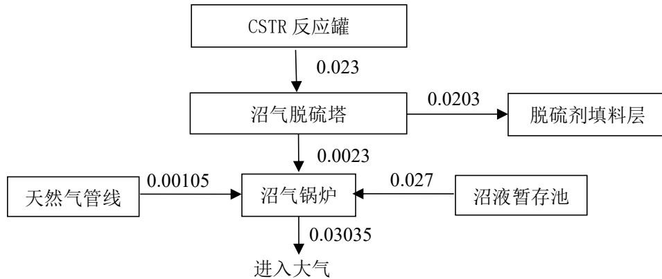
图 3.12-5 本项目沼气锅炉硫平衡图 单位：t
