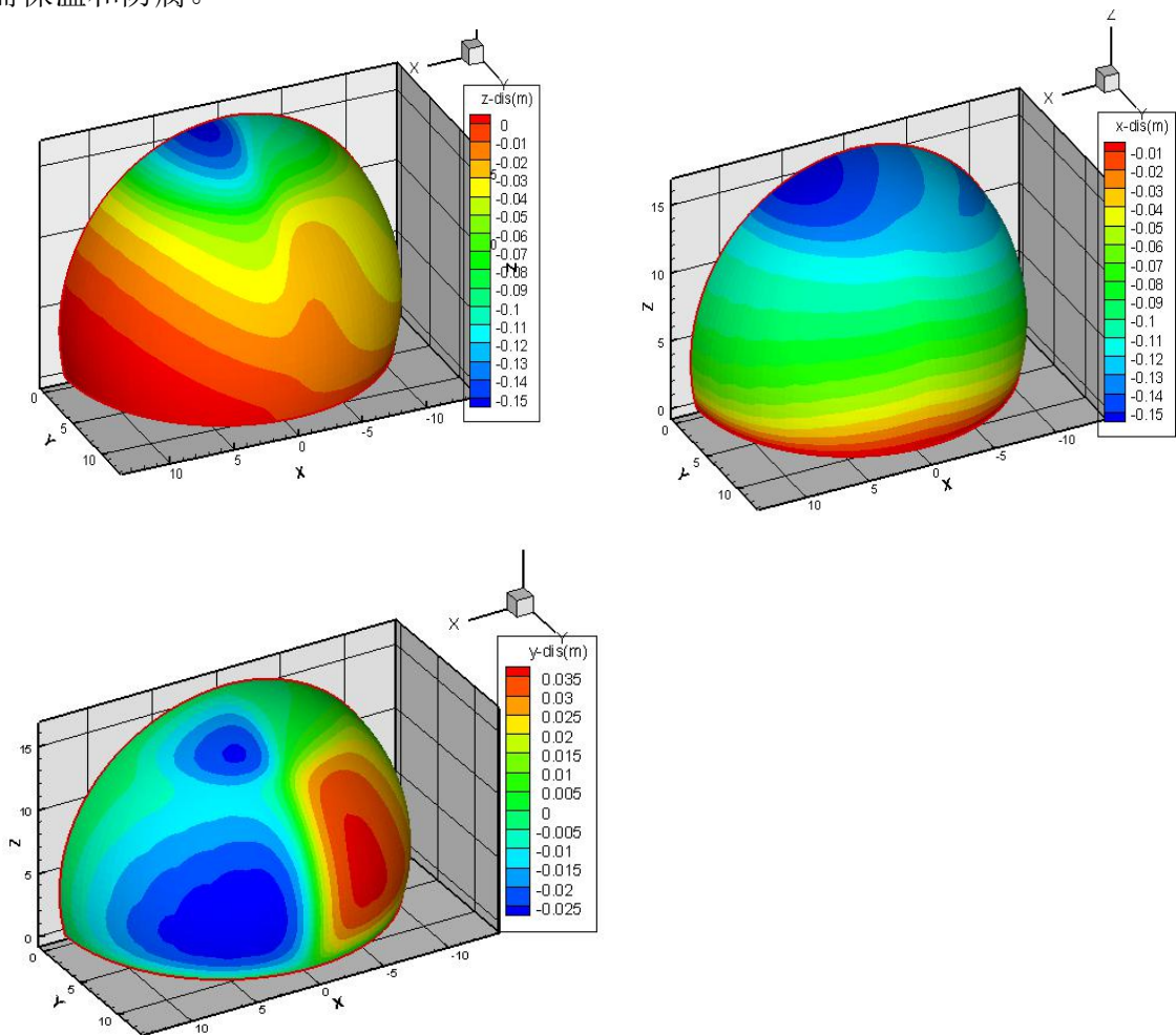
图 3.4-1 气柜受力分析图
