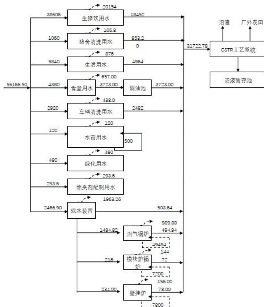
图 3.12-3 本项目水平衡图 单位: m³/a
