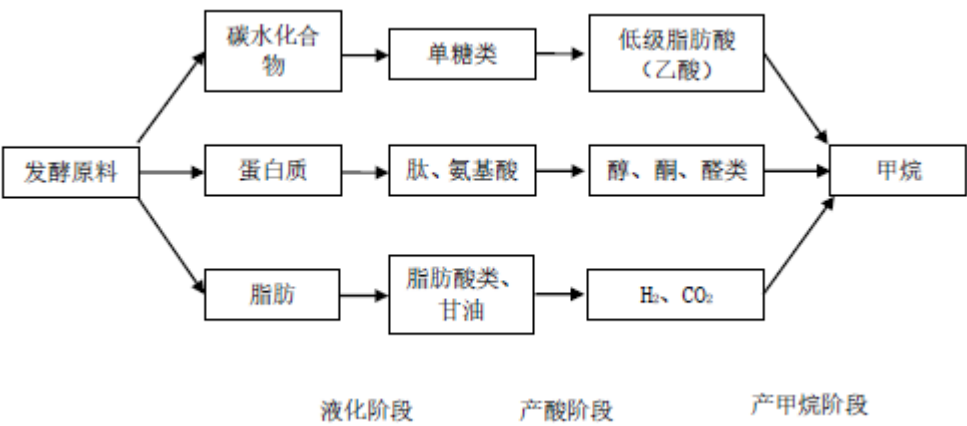
图 3.4-1 沼气发酵原理流程图
