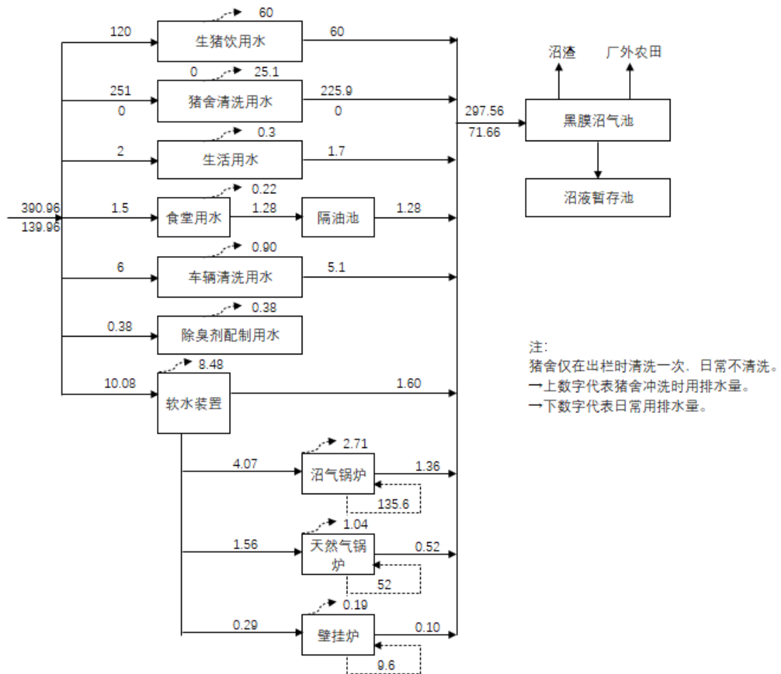
图 3.12-2 本项目其他季节（245 天）水平衡图 单位：m 3 /d
