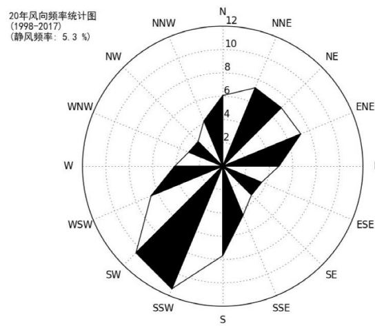
图 5.2-1 沈阳风向玫瑰图（静风频率 5.3%）
